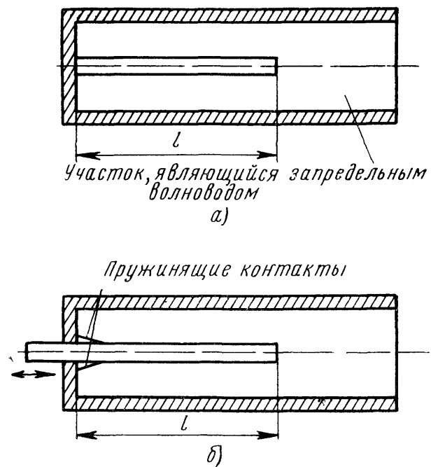
Рис. 10.4. Особенности конструктивного выполнения четвертьволновых резонаторов
