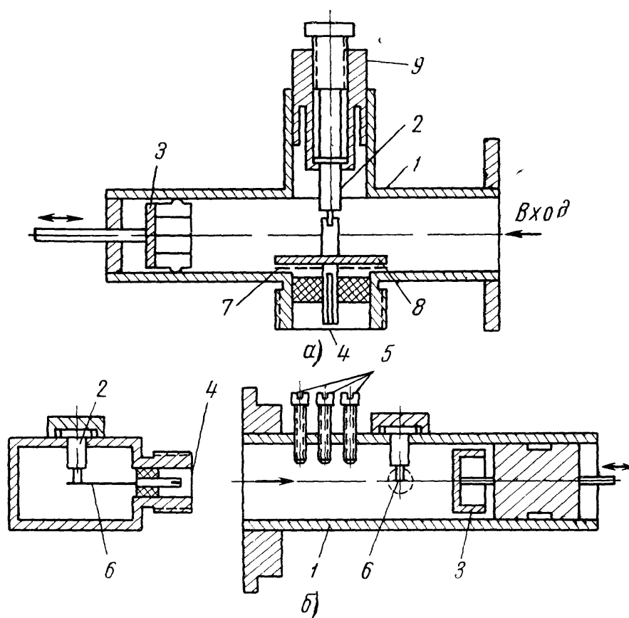
Рис. 8.25. Схема устройства двух настраиваемых волноводных детекторных головок
