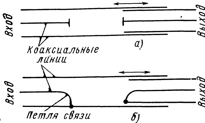
Рис. 5.19. Принцип устройства предельных ослабителей а — ослабитель на волне типа E_{01} ; б — ослабитель на волне типа H_{11}
