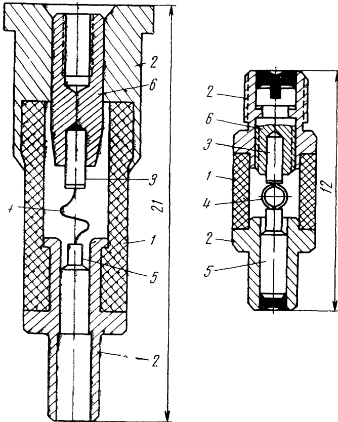
Рис. 7.7. Устройство двух типичных кристаллических детекторов сантиметрового диапазона
