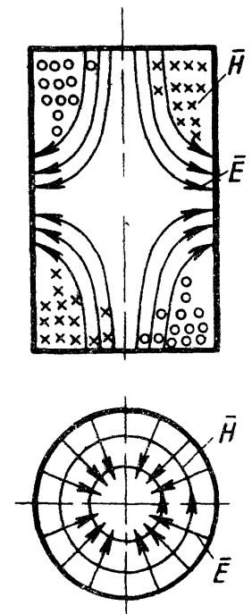
Рис. 10.21. Структура поля в цилиндрическом резонаторе при виде колебаний E_{011}
