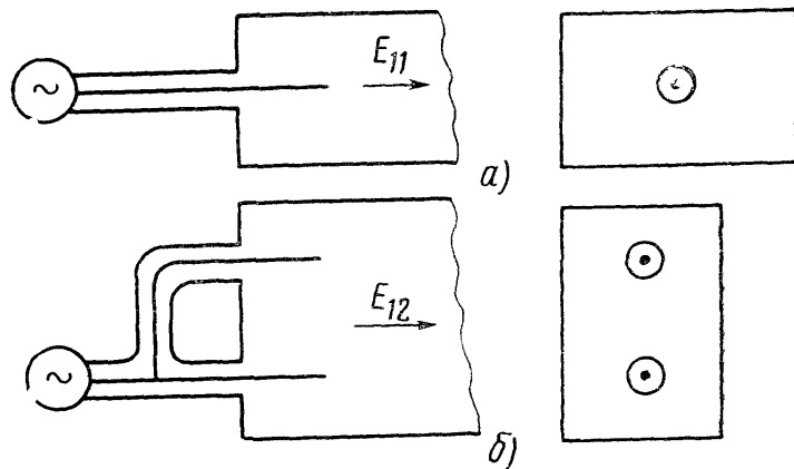
Рис 5.2 Возбуждение волн типа ТМ в прямоугольном волноводе с помощью электрического диполя
