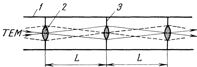
Рис. 12.5. Линзовый лучевой волновод
