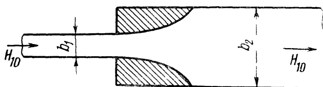
Рис. 7.34. Экспоненциальный трансформатор в прямоугольном волноводе
