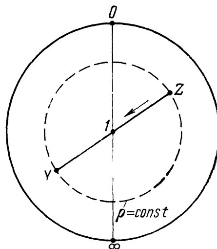
Рис. 7.22. Нахождение проводимости по заданному полному сопротивлению
