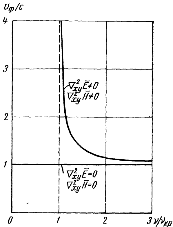
Рис. 2.3. Зависимость фазовой скорости волны в передающей линии от частоты в случае вакуумного наполнения ( \epsilon = \mu = 1 )
