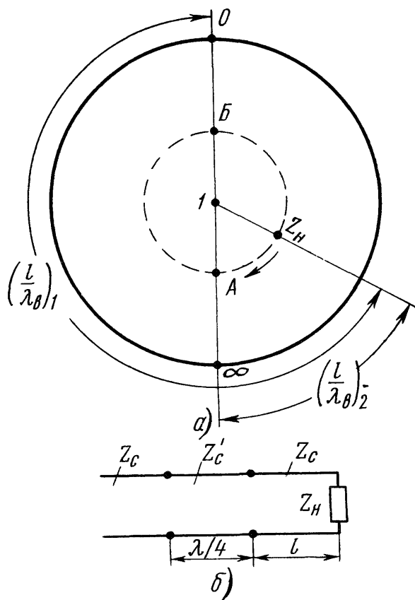
Рис. 7.27. Применение четвертьволнового трансформатора для согласования комплексной нагрузки
