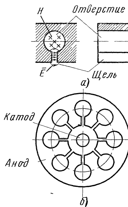
Рис. 10.30. Одиночный резонатор типа «щель — отверстие» (а) и свернутый в кольцо многорезонаторный анодный блок магнетрона (б). Показана структура электрического и магнитного полей в одиночном резонаторе
