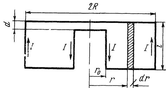
Рис. 10.26. Тороидальный полый резонатор
