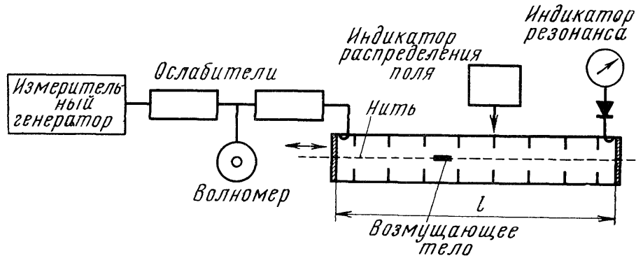
Рис. 11.30. Блок-схема резонансных измерений параметров замедляющих систем
