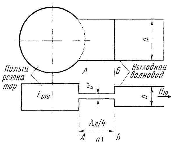
Рис. 10.38. Связь цилиндрического резонатора с прямоугольным волноводом через четвертьволновый трансформатор
