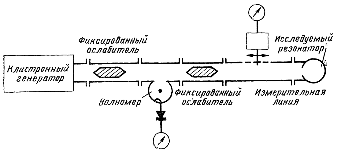
Рис. 10.40. Блок-схема волноводной установки с измерительной линией для измерения параметров полого резонатора по методу двухполюсника
