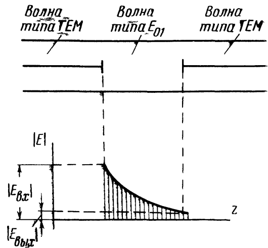
Рис. 5.20. Принцип действия предельного ослабителя
