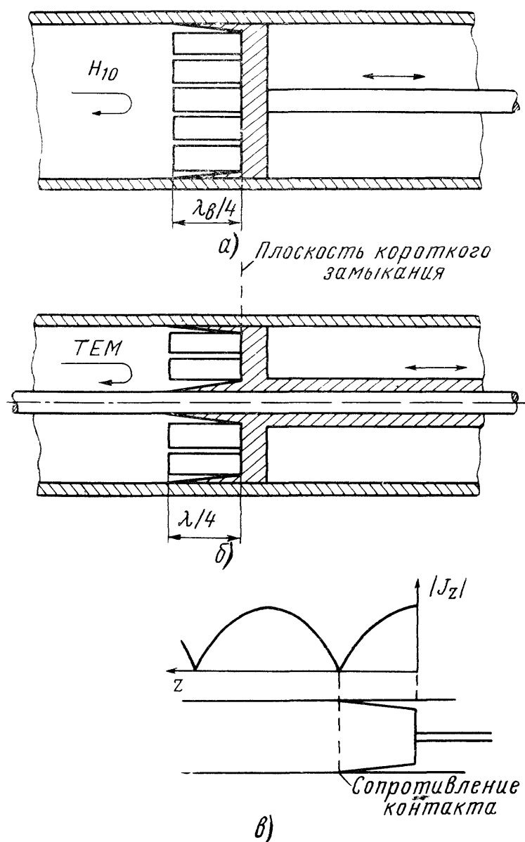
Рис. 8.7. Короткозамыкающие поршни с пружинящими контактами
