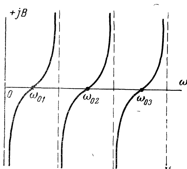
Рис. 9.4. Изменение реактивной проводимости отрезка короткозамкнутой длинной линии
