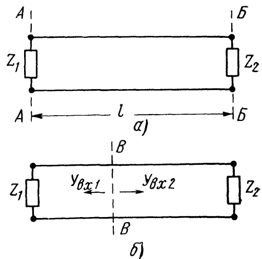
Рис. 10.2. Обобщенная эквивалентная схема резонаторов, изображенных на рис. 10.1
