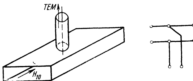
Рис. 6.27. Смешанный коаксиально-волноводный тройник со штырем связи и его упрощенная эквивалентная схема
