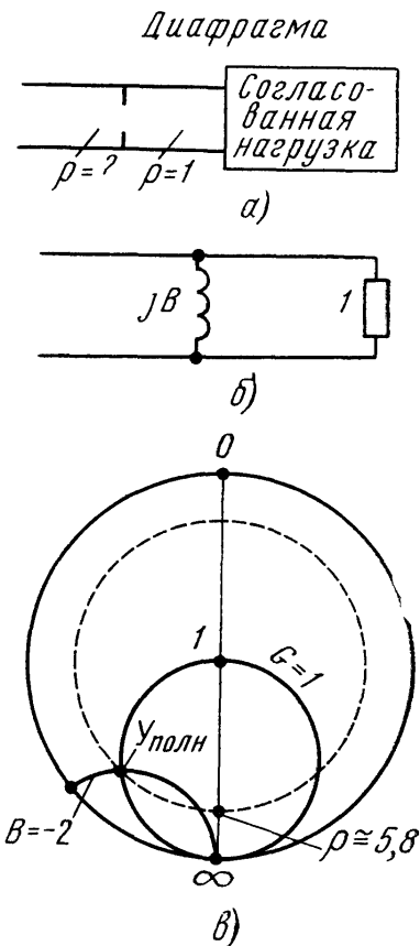
Рис. 7.18. Расчет КСВ при включении в волновод индуктивной диафрагмы с заданной величиной B = -2
