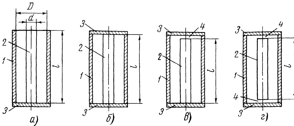
Рис. 10.1. Полые резонаторы, рассматриваемые как отрезки коаксиальных линий
