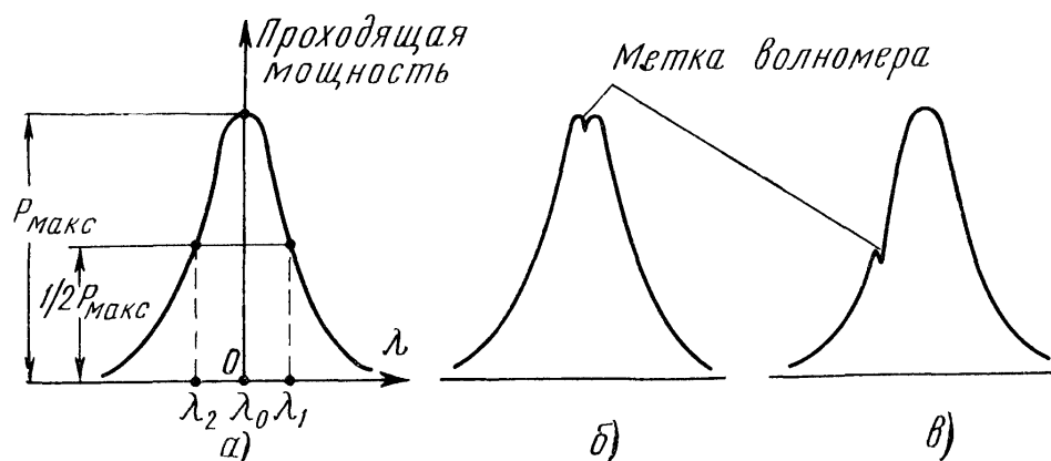
Рис. 10.45. К определению длин волн \lambda_0 , \lambda_1 и \lambda_2 по осциллограмме резонансной кривой в схеме, изображенной на рис. 10.44
