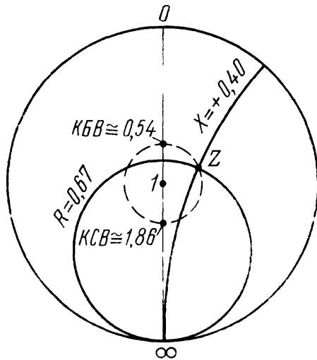
Рис. 7.17. Нахождение на круговой диаграмме точки Z_n = 50 + j30 (о.м.) при Z_c = 75 о.м. Пунктиром проведена окружность постоянного КСВ, соответствующего рассматриваемой нагрузке
