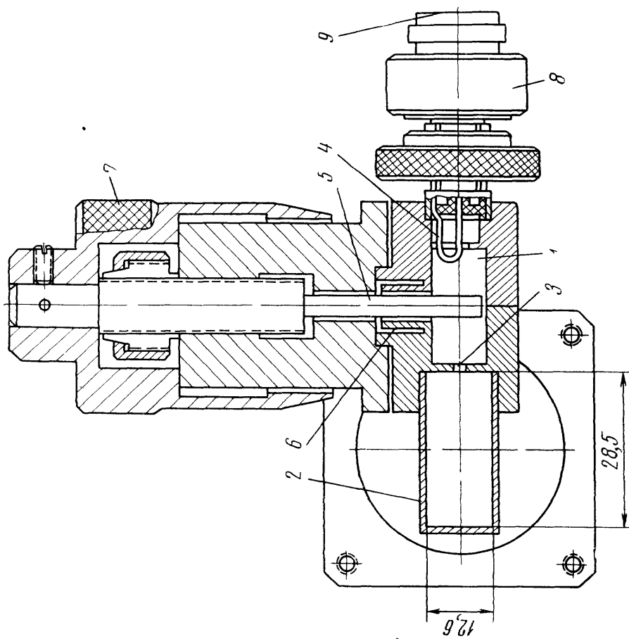
Рис. 10.36. Устройство проходного резонансного волномера 3-см диапазона, имеющего цилиндрический резонатор с укорачивающей емкостью (вид колебаний E_{010} ). Связь резонатора с волноводом осуществляется через отверстие, связь с детектором — через петлю
