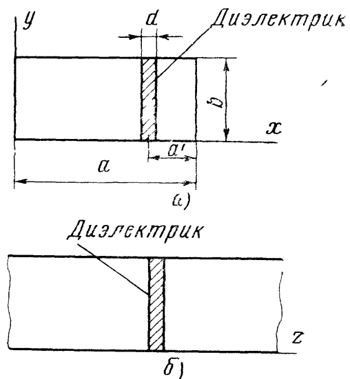
Рис. 5.10. Волновод с частичным диэлектрическим наполнением (случаи продольного и поперечного расположения диэлектрической пластины)
