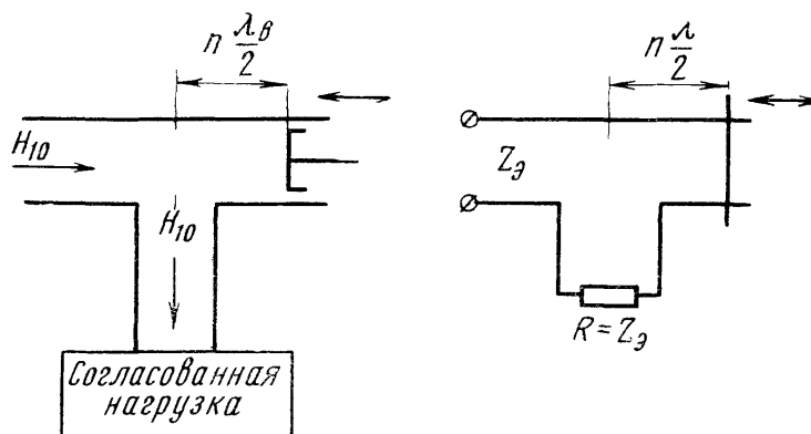
Рис. 6.25. Применение короткозамыкающего поршня и согласованной нагрузки для проверки свойств волноводного Е-тройника
