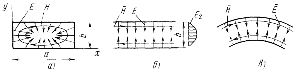
Рис. 4.10. Получение волны типа E_{01} в коаксиальном волноводе из волны типа E_{11} в прямоугольном волноводе
