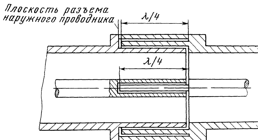
Рис 8.6 Дроссельное сочленение жесткой коаксиальной линии
