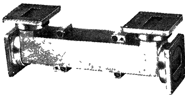
Рис. 8.43. Внешний вид направленного ответвителя 3-см диапазона
