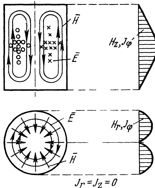
Рис 10.23. Структура и эшюры поля и тока в стенках цилиндрического резонатора при виде колебаний H_{011}
