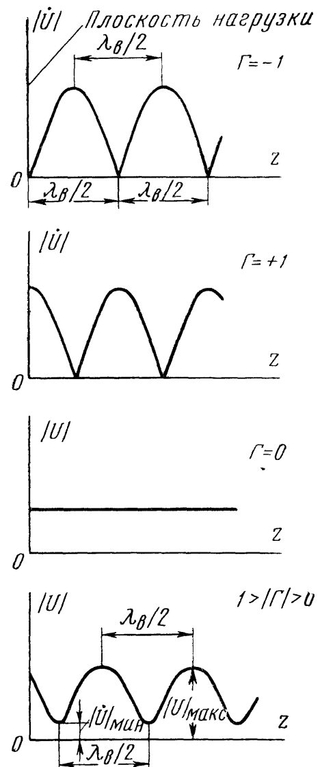
Рис. 7.3. Различные режимы распределения напряжения в передающей линии без потерь, отличающиеся величиной коэффициента отражения
