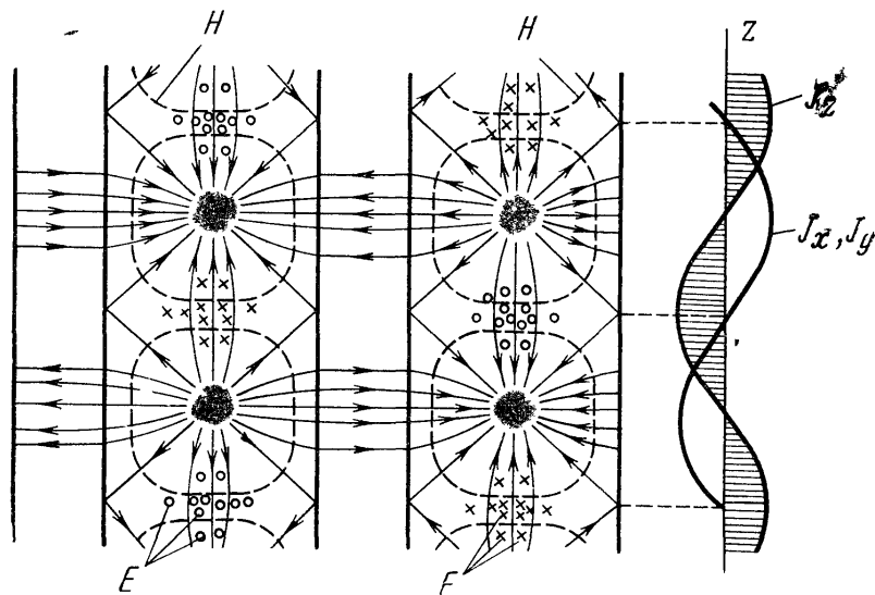
Рис. 3.19. Распределение поверхностных токов в прямоугольном волновоеде при волне типа H_{10} и расположение электрических и магнитных силовых линий бегущей волны
