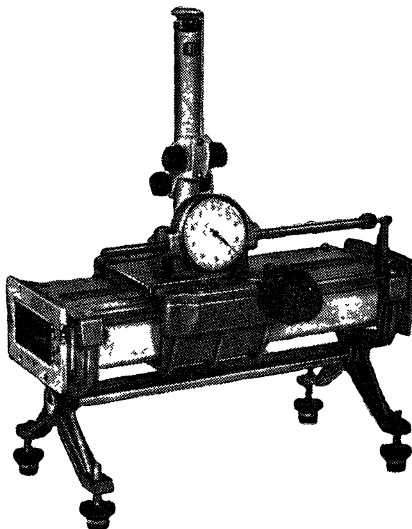
Рис. 8.35. Внешний вид волноводной измерительной линии 10-см диапазона
