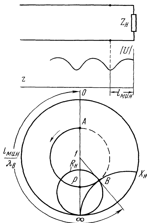
Рис. 7.20. Определение сопротивления нагрузки по измеренным величинам \rho и l_{\text{мин}}/\lambda_{\text{в}}
