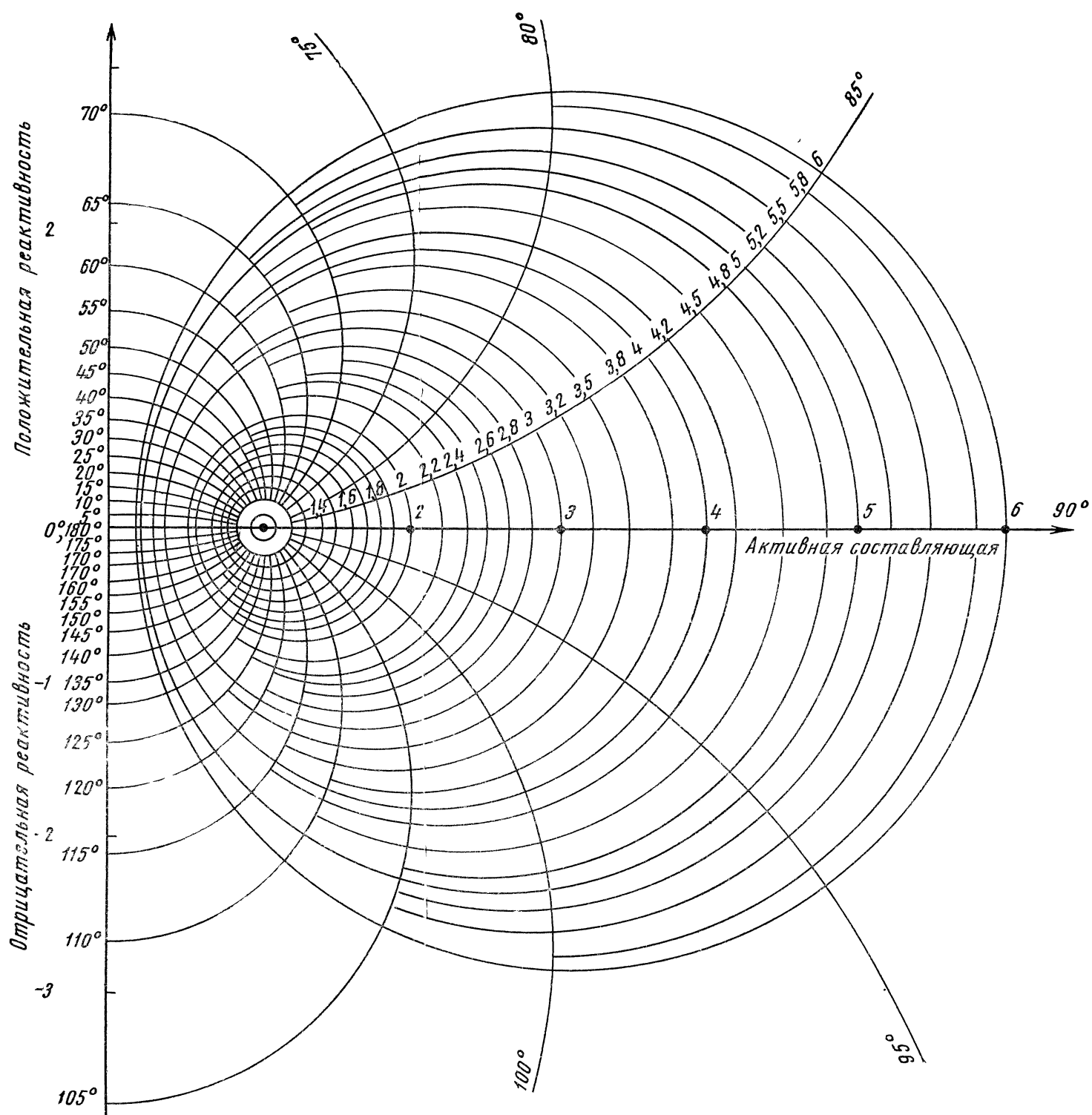
Рис. 7.16. Круговая диаграмма полных сопротивлений и проводимостей в прямоугольной системе координат
