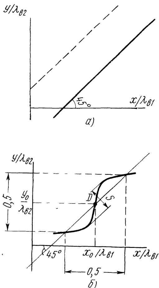
Рис. 7.11. Зависимость положения минимума стоячей волны во входной линии от положения поршня в выходной линии для схемы, показанной на рис. 7.10
