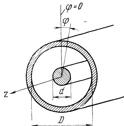
Рис. 4.9. Коаксиальный волновод
