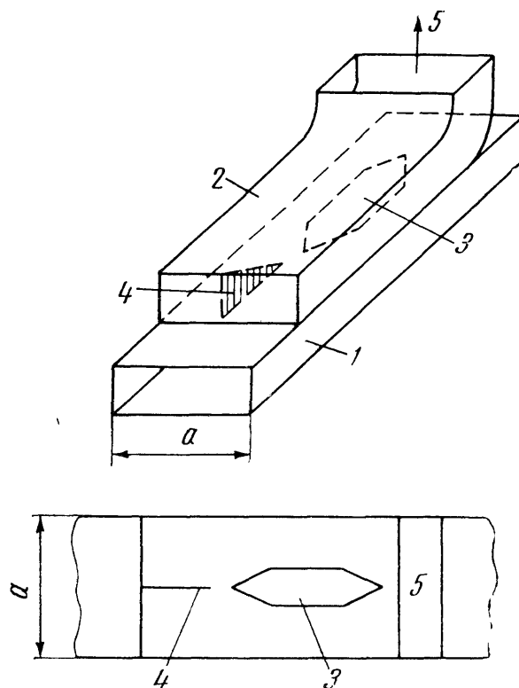
Рис. 8.42. Схема устройства волноводного направленного ответвителя с длинной щелью
