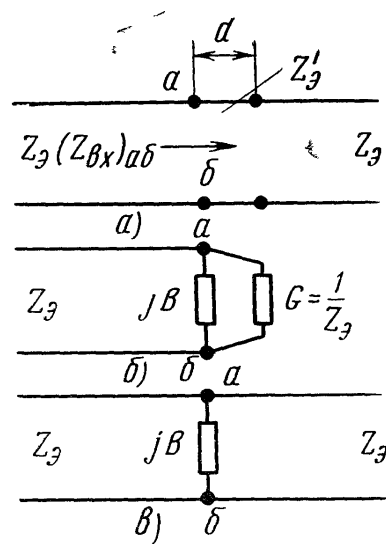
Рис. 6.9. Преобразования эквивалентной схемы тонкой диафрагмы в волноводе
