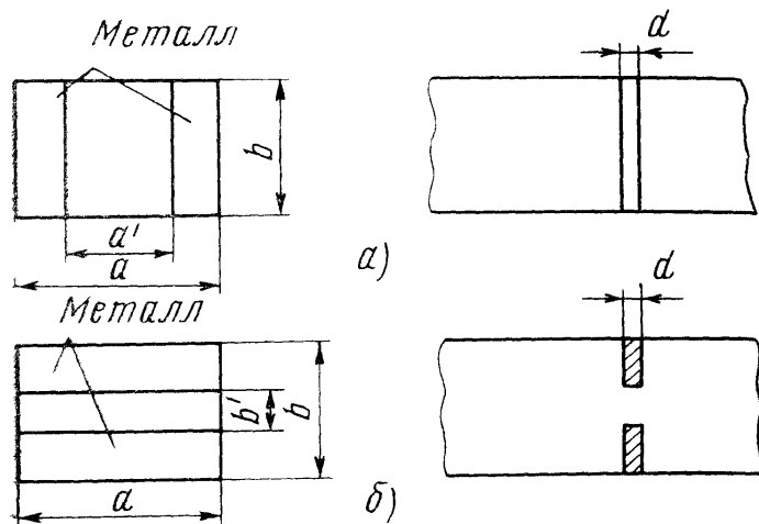
Рис. 6.8. Простейшие симметричные диафрагмы в прямоугольном волноводе
