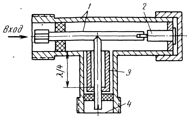
Рис. 8.26. Схема устройства ненастраиваемой коаксиальной детекторной головки
