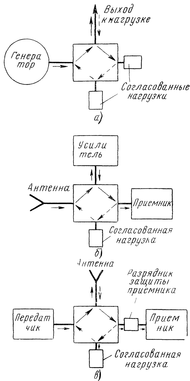
Рис. 8.57. Примеры применения циркуляторов
