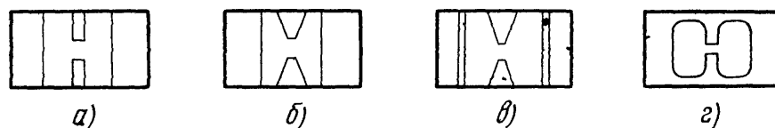
Рис. 6.38. Варианты конструкций резонансных зазоров
