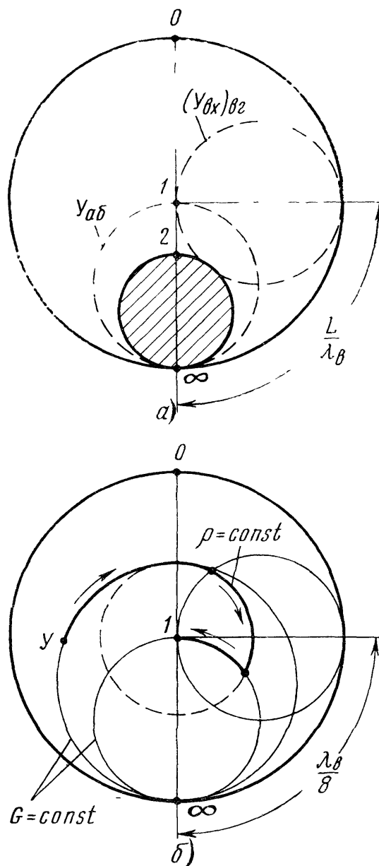
Рис. 7.31. Объяснение действия двухшлейфового трансформатора на диаграмме полных проводимостей
