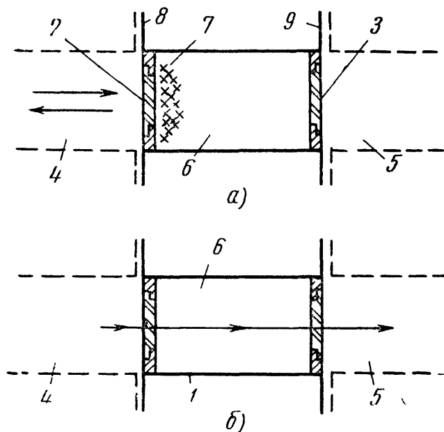
Рис 6.18 Использование резонансного окна в качестве разрядного промежутка
