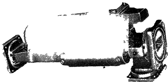
Рис. 8.54. Внешний вид ферритового фазового циркулятора
