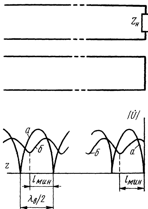
Рис. 7.21. Опыт короткого замыкания нагрузки для определения l_{\text{мин}}
