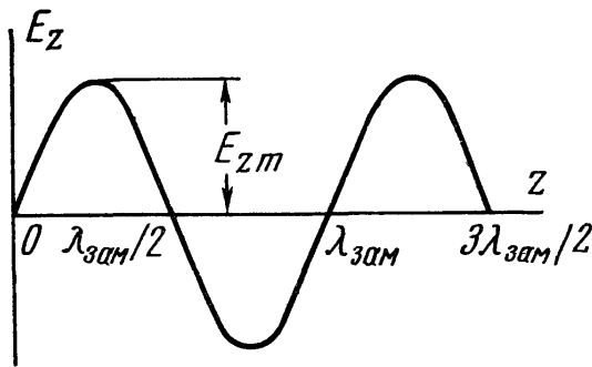
Рис. 11.6. Эпюра продольной составляющей замедленной волны типа ТМ
