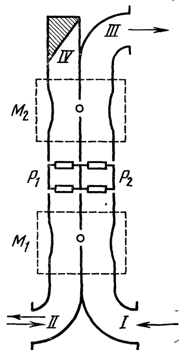
Рис. 8.51. Схема балансного антенного переключателя, использующего два щелевых моста и два разрядника защиты приемника или один сдвоенный разрядник с общей вакуумной оболочкой
