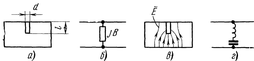
Рис. 6.36. Штырь в прямоугольном волноводе и его эквивалентные схемы
