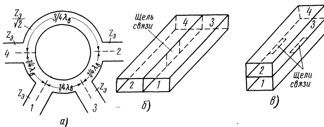
Рис. 8.48. Волноводные мостовые соединения
