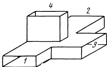
Рис. 6.34. Двойной волноводный тройник
