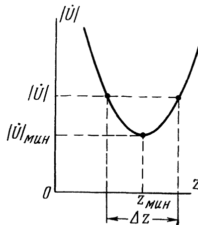
Рис. 7.9. К измерению КСВ по ширине узла стоячей волны
