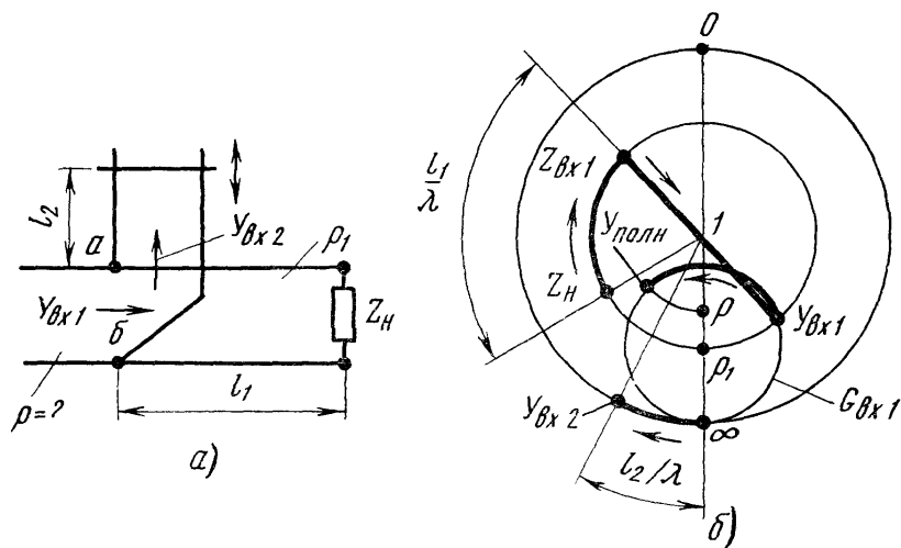
Рис. 7.23. Нахождение КСВ на входе разветвленной цепи
