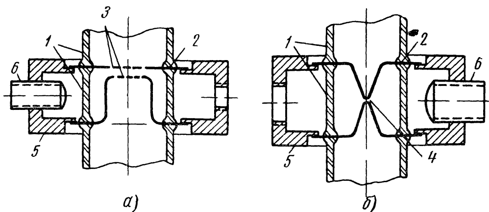
Рис 10.29 Полые резонаторы с индуктивной настройкой в невакуумной части, применяемые в отражательных клистронах (а) и в высокودобротных резонансных разрядниках (б)
