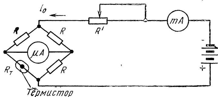
Рис. 8.34. Принципиальная схема термисторного моста
