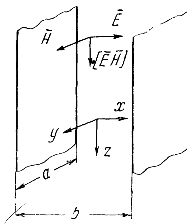
Рис. 6.4. К расчету характеристического сопротивления ленточной линии
