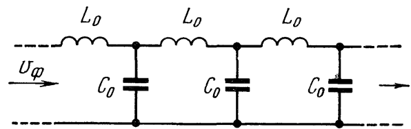
Рис. 11.1. Низкочастотная линия задержки, обеспечивающая v_{\phi} < c
