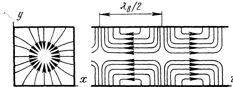
Рис. 3.4. Структура электрического поля в прямоугольном волноводе при волне типа E_{11}
