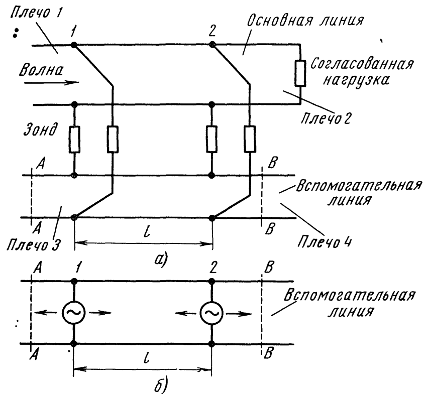
Рис. 8.37. Принцип действия направленного ответвителя с двумя зондами
