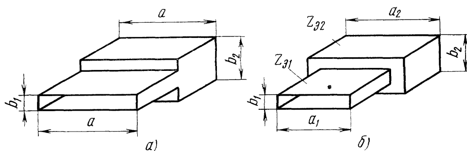
Рис. 6.5. Неоднородности типа ступеньки в прямоугольном волноводе
