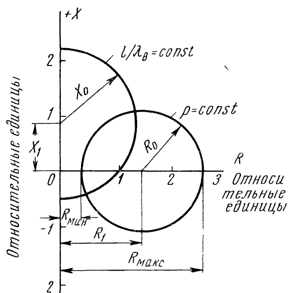
Рис. 7.15. Окружности постоянных значений КСВ и постоянной фазы на плоскости полных сопротивлений в прямоугольной системе координат
