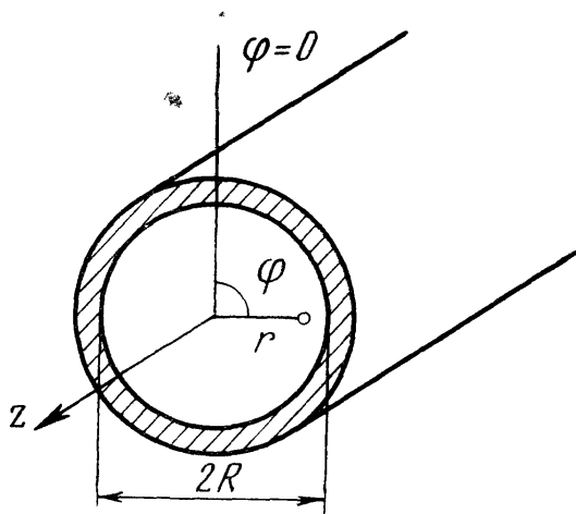
Рис. 4.1. Волновод круглого сечения
