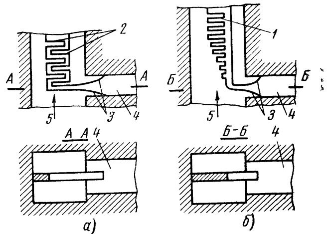
Рис 11.28 Плавные переходы от замедляющих систем типа встречных штырей (а) и гребенки (б) к волноводу прямоугольного сечения в миллиметровом диапазоне волн 1 — гребенка, 2 — зубцы встречноштыревой системы, 3 — экспоненциальные выступы, 4 — прямоугольный волновод 5 — электронный пучок
