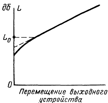
Рис. 8.15. Типичная рабочая характеристика предельного ослабителя
