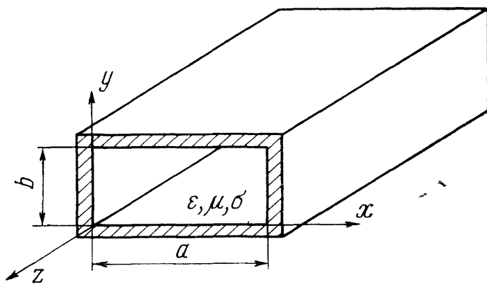
Рис. 3.1. Волновод прямоугольного сечения
