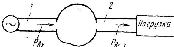
Рис. 9.8. Проходное включение полового резонатора (схема четырехполюсника)
