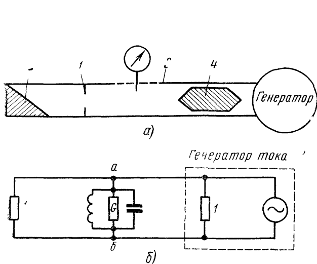
Рис. 9.3. Резонансное окно, включенное поперек волновода для измерения полной проводимости, и соответствующая эквивалентная схема
