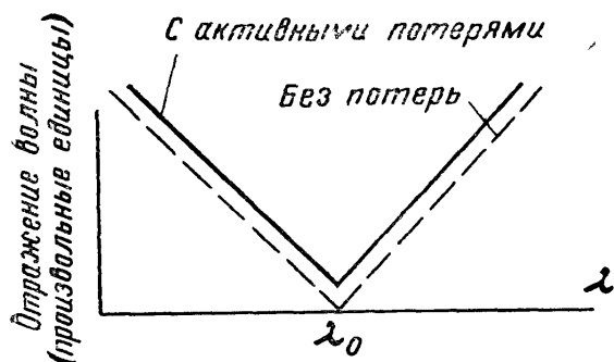
Рис. 6.15. Характер отражения волны от резонансного окна в волноводе
