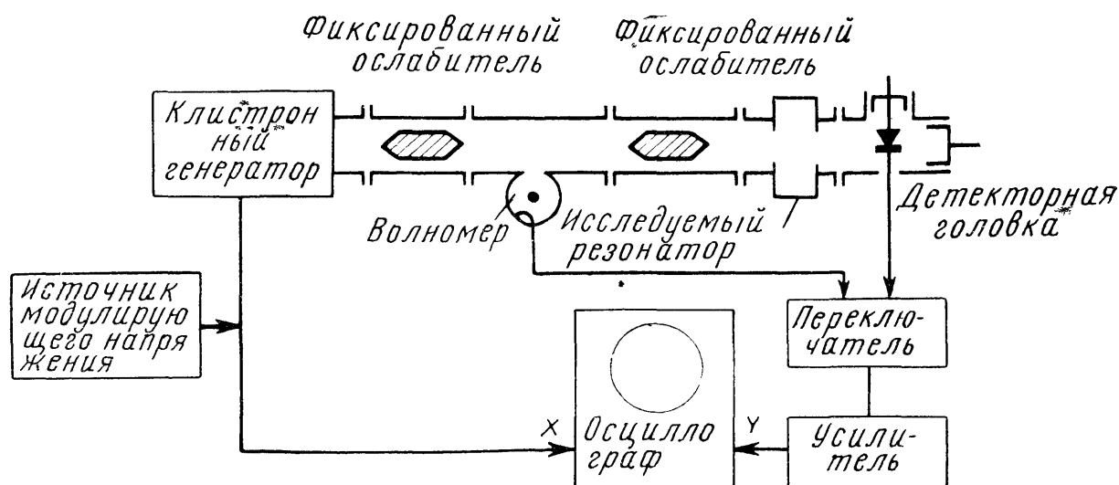
Рис. 10.44. Блок-схема волноводной установки для осциллографического измерения параметров полых резонаторов с двумя элементами связи
