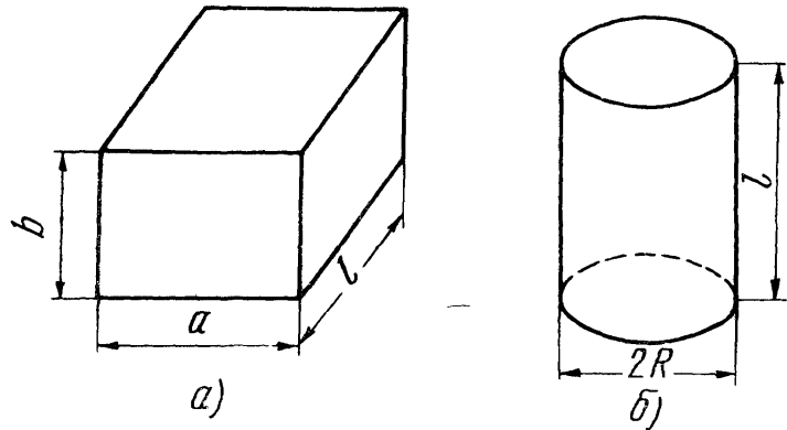
Рис. 10.16. Призматический и цилиндрический полые резонаторы
