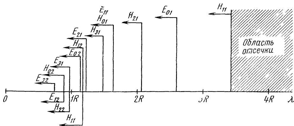
Рис. 4.7. Критические длины волн волновода круглого сечения
