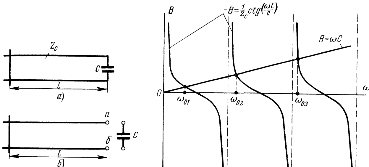
Рис. 10.8. Эквивалентная схема резонатора типа коаксиальной линии, нагруженной на емкость
