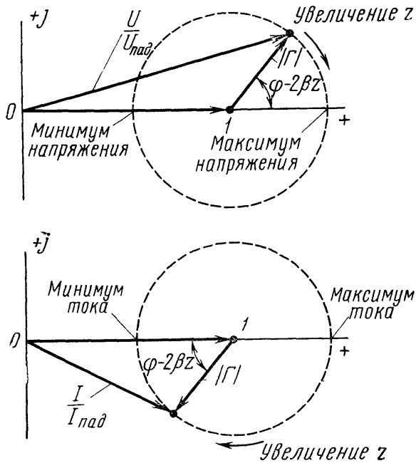
Рис. 7.1. Векторные диаграммы, иллюстрирующие уравнения (7.9) и (7.10)
