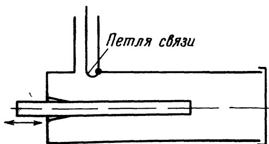
Рис. 10.14. Связь четвертьволнового резонатора с коаксиальной линией при помощи петли
