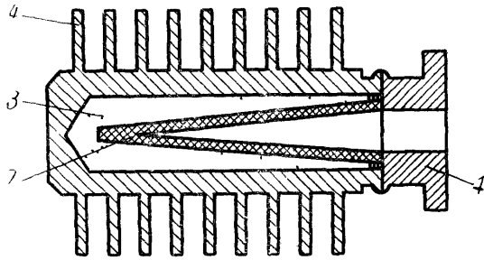
Рис. 8.11. Устройство согласованной волноводной нагрузки высокого уровня мощности
