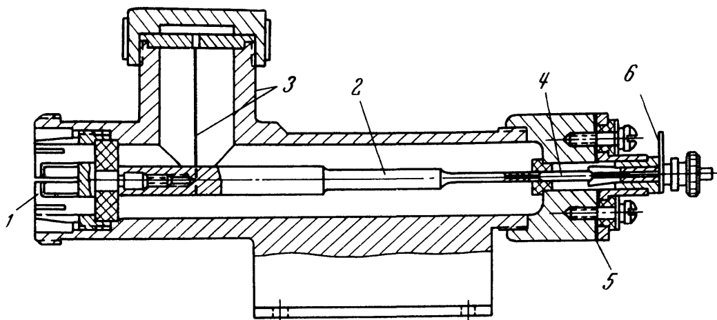
Рис. 8.33. Устройство широкополосной коаксиальной термисторной головки:
