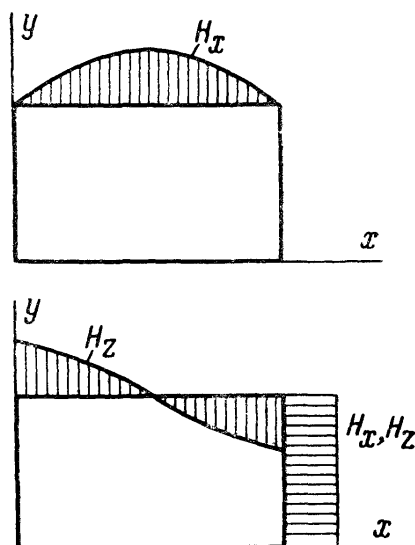
Рис. 3.8. Эпюры магнитного поля в поперечном сечении волновода при волне типа H_{10}
