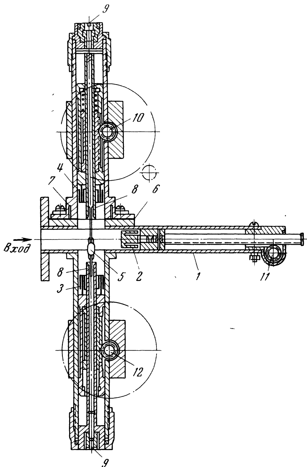
Рис. 8.32. Пример устройства волноводной настраиваемой термисторной головки
