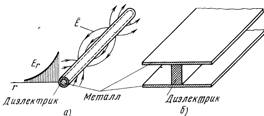
Рис. 5.17. Волноводные линии:
