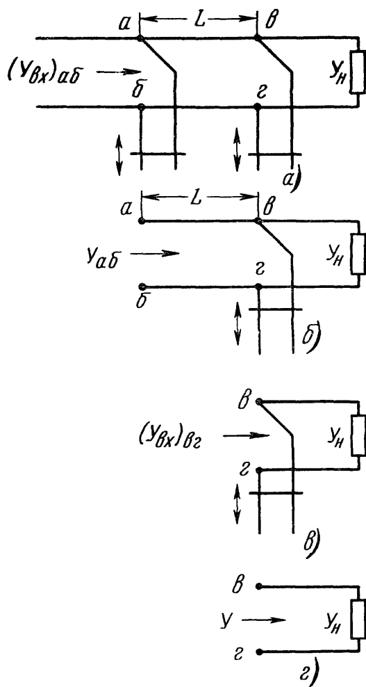
Рис. 7.30. Двухшлейфовый трансформатор полных сопротивлений
