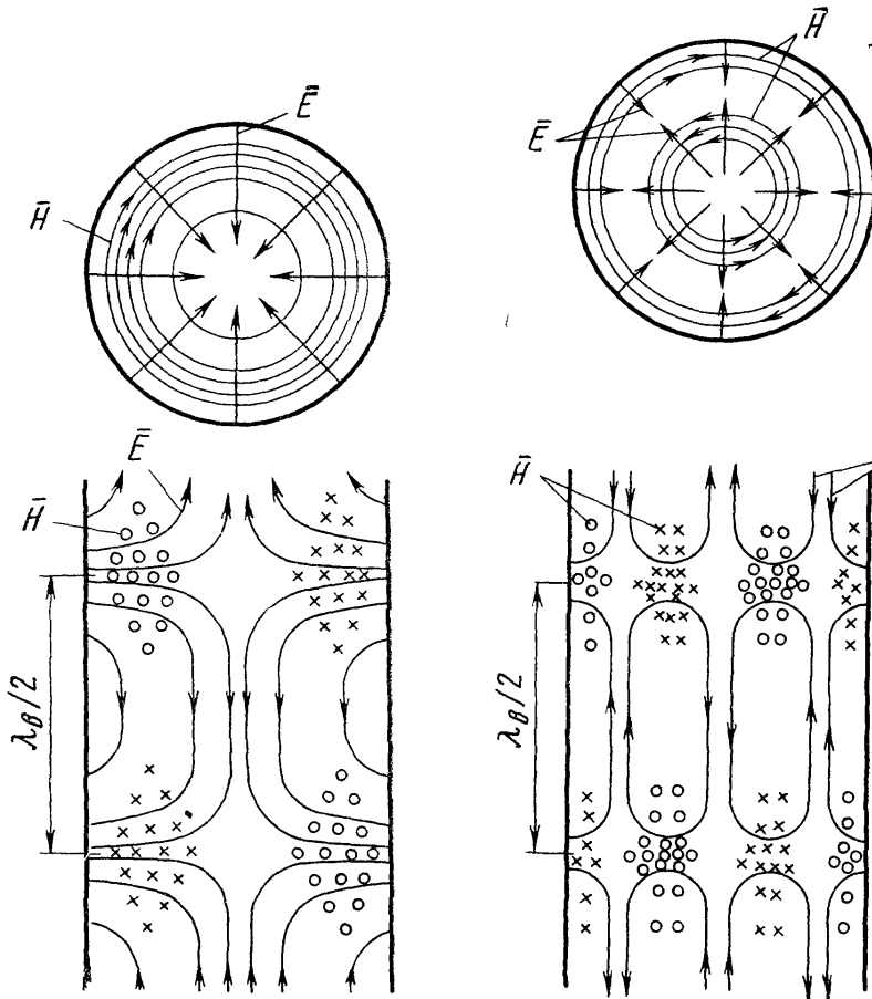
Рис. 4.3. Структура электрического и магнитного полей при бегущей волне типа E_{01} в круглом волноводе
