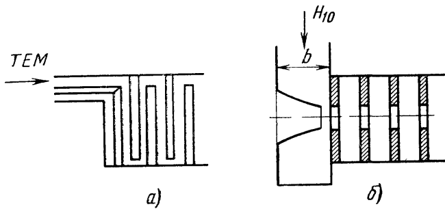
Рис 11.27 Связь замедляющей системы типа встречных штырей с коаксиальной линией (а) и системы типа круглого диафрагмированного волновода со стандартным волноводом прямоугольного сечения (б)
