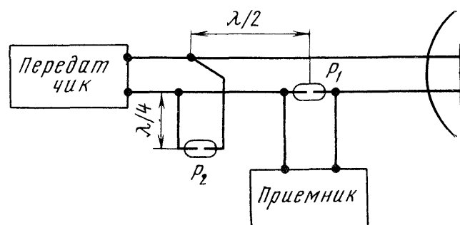
Рис. 6.32. Схема ответвительного антенного переключателя с параллельным включением разрядника блокировки передатчика и последовательным включением разрядника защиты приемника
