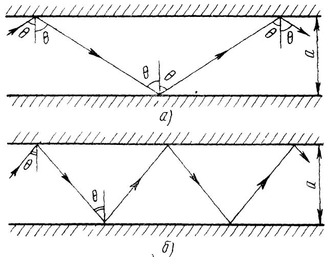
Рис. 2.6. Зигзагообразное распространение волны типа ТЕМ между параллельными проводящими поверхностями. В случае (а) отношение \frac{\lambda}{\lambda_{кр}} меньше, чем в случае (б)
