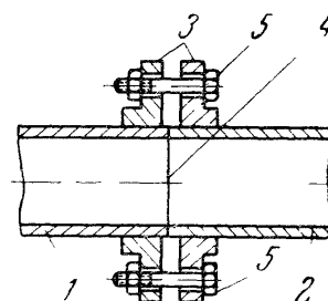
Рис. 8.1. Контактное соединение волноводов
