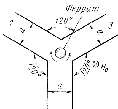
Рис. 8.56. Схема волнового Y-циркулятора
