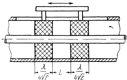
Рис. 7.33. Двухшайбовый диэлектрический трансформатор в коаксиальной линии
