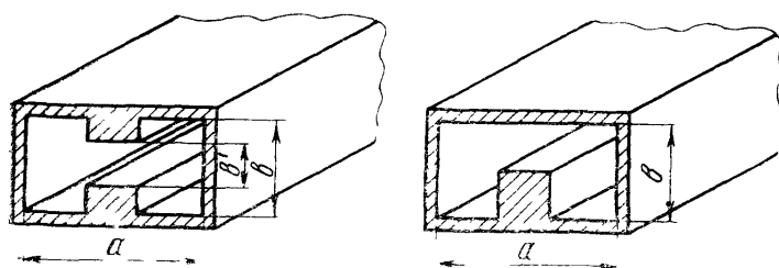
Рис. 5.12 Ребристые волноводы Н- и П-образного сечений
