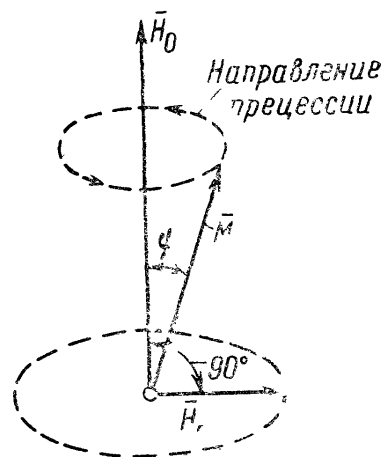
Рис. 8.17. Прецессия магнитного момента электрона в постоянном магнитном поле
