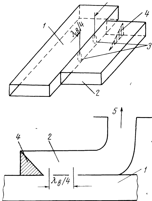
Рис. 8.41. Схема устройства двухдырочного направленного ответвителя
