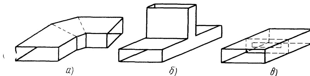
Рис. 6.1. Примеры неоднородностей в прямоугольном волноводе
