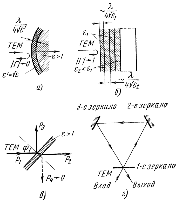
Рис. 12.4. К рассмотрению аналогии между оптическими устройствами и элементами техники СВЧ.
