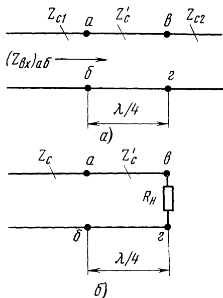
Рис. 7.25. Применение четвертьволнового трансформатора
