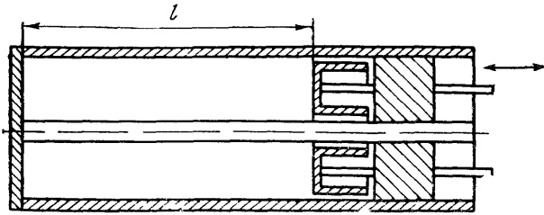
Рис. 10.6. Перестройка коаксиального полуволнового резонатора с помощью передвижного дроссельного поршня
