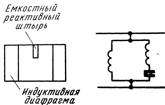
Рис. 6.37. Устройство и эквивалентная схема резонансного зазора
