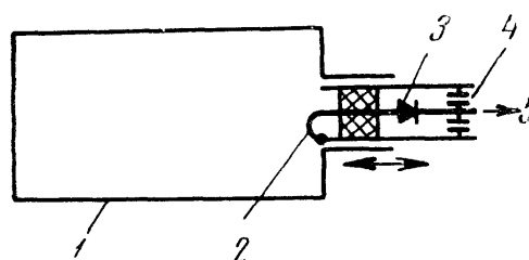
Рис. 8.28. Схема включения петлевого индикатора с кристаллическим детектором
