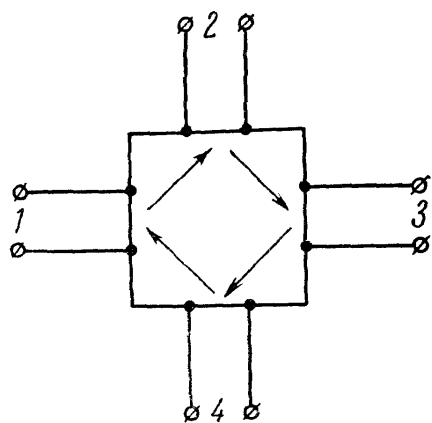
Рис. 8.52. Передача энергии между плечами идеального восьмипольного циркулятора
