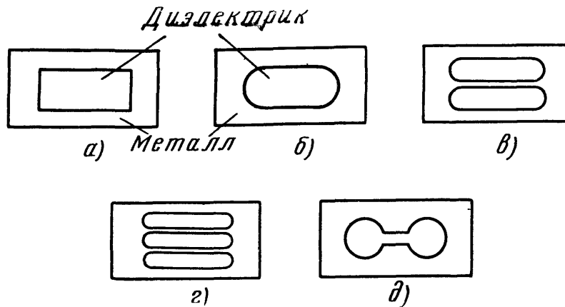
Рис. 6.13. Примеры окон в прямоугольном волноводе
