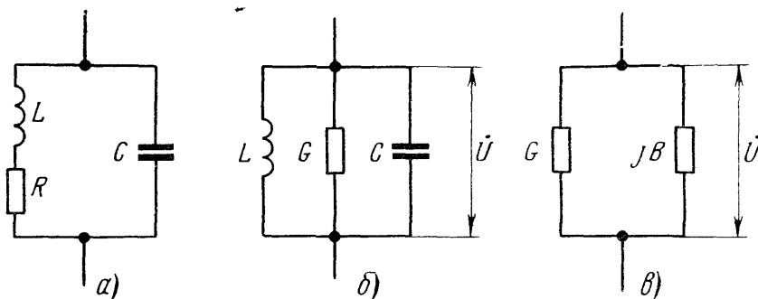
Рис. 9.1. Варианты эквивалентной схемы полого резонатора
