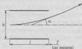
Рис. 1.8. Плоскопараллельные отклоняющие пластины
