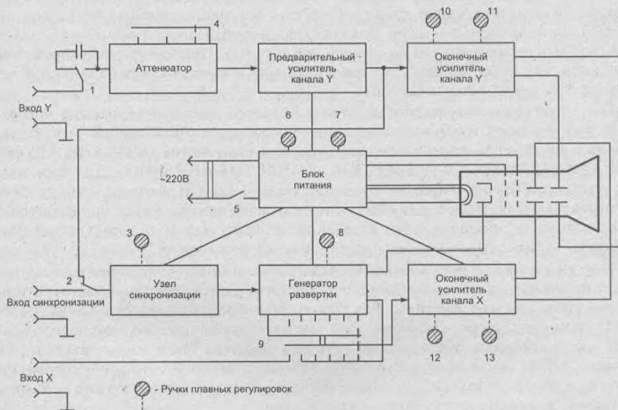
Рис. 1.12. Типовая функциональная схема электронного осциллографа
