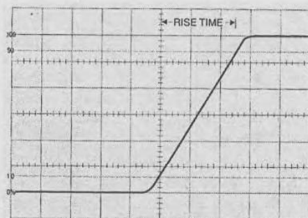
Рис. 5.22. Пример измерения времени нарастания импульсного перепада
