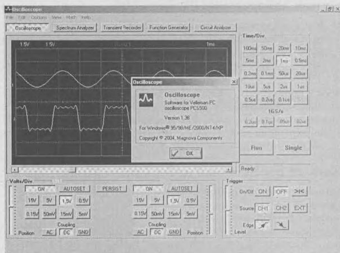
Рис. 4.19. Окно обновленного виртуального осциллографа PCS500
