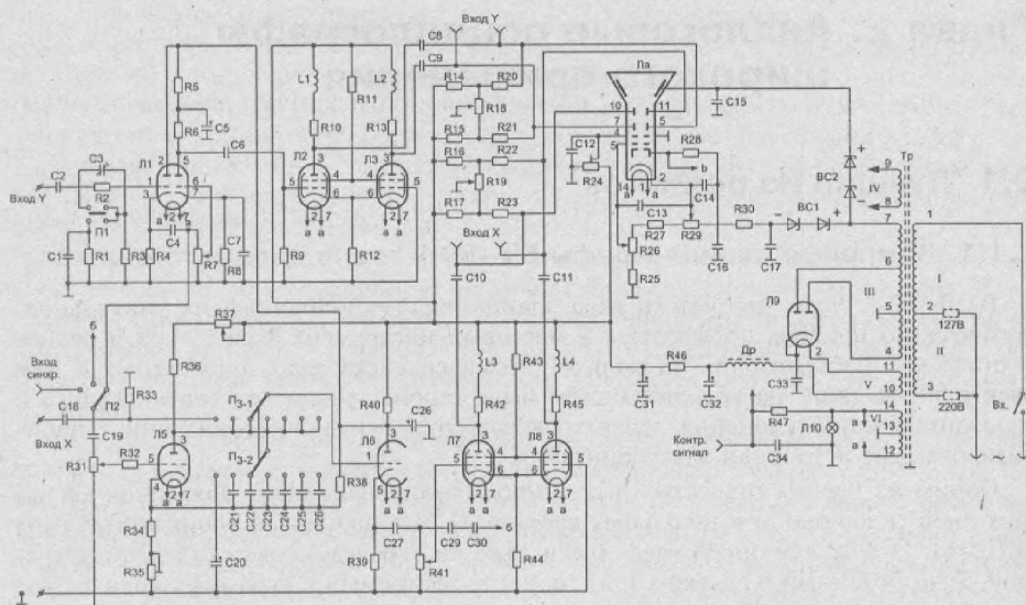
Рис. 2.1. Принципиальная схема осциллографа ОЗШ-61
