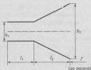
Рис. 1.9. Отклоняющие пластины с одним изгибом
