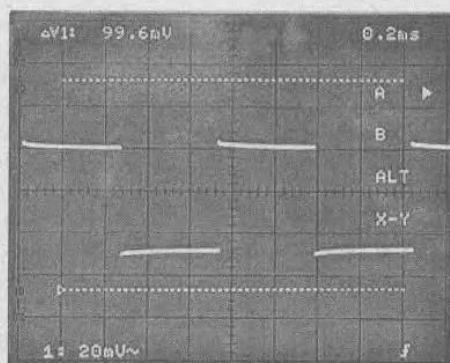
Рис. 5.42. Экран осциллографа с горизонтальными курсорами
