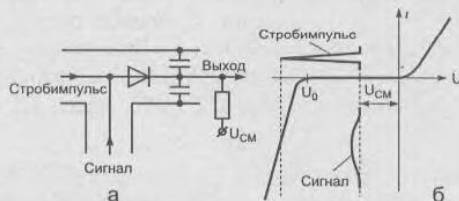
Рис. 3.6. Схема стробирования на скоростном лавинном диоде
