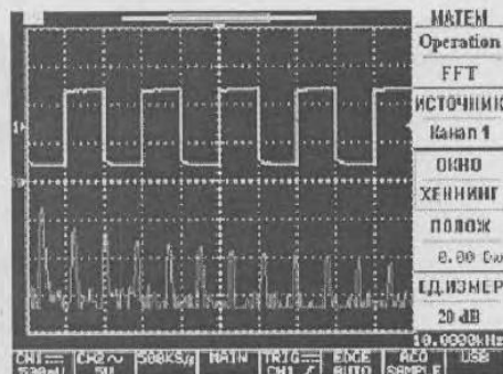
Рис. 5.67. Осциллограммы меандра и его спектра
