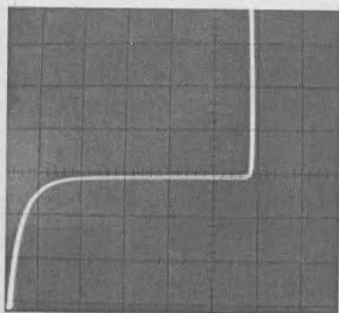
Рис. 5.31. Вольт-амперная характеристика кремниевого стабилитрона
