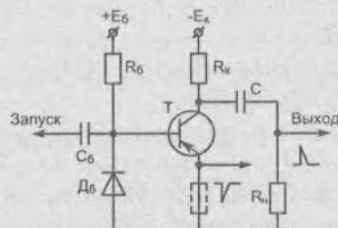
Рис. 3.4. Генератор коротких импульсов на лавинном транзисторе
