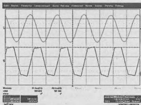
Рис. 5.46. Осциллограммы сигнала 500 МГц, полученные осциллографом LeCroy WS-452 при интерполяции функцией \sin(x)/x (сверху) и при линейной интерполяции (снизу)
