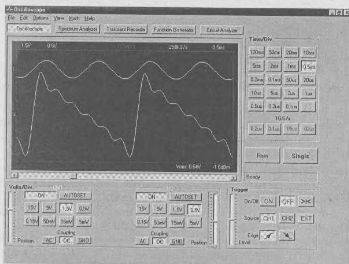
Рис. 4.5. Окно виртуального осциллографа PCS500 в режиме осциллографа
