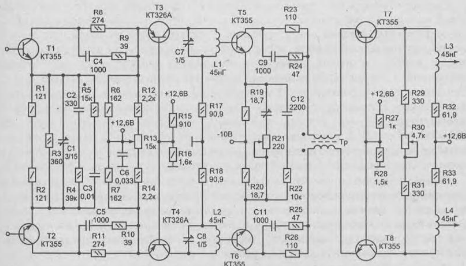
Рис. 1.18. Предварительный усилитель осциллографа С1-71
