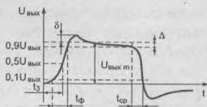
Рис. 1.16. Временные характеристики реальных импульсных сигналов
