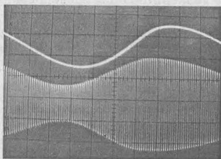
Рис. 5.35. Одновременное наблюдение полного периода модулирующего сигнала и 100 периодов модулированного сигнала
