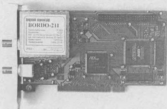
Рис. 4.31. PCI плата одноканального 120-мегагерцевого осциллографа B-211
