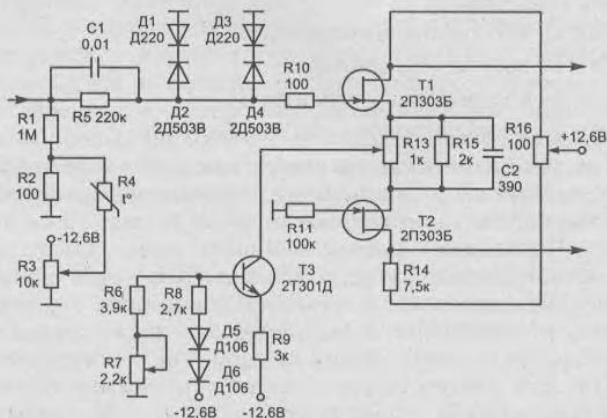
Рис. 1.17. Входной каскад усилителя У осциллографа С1-68
