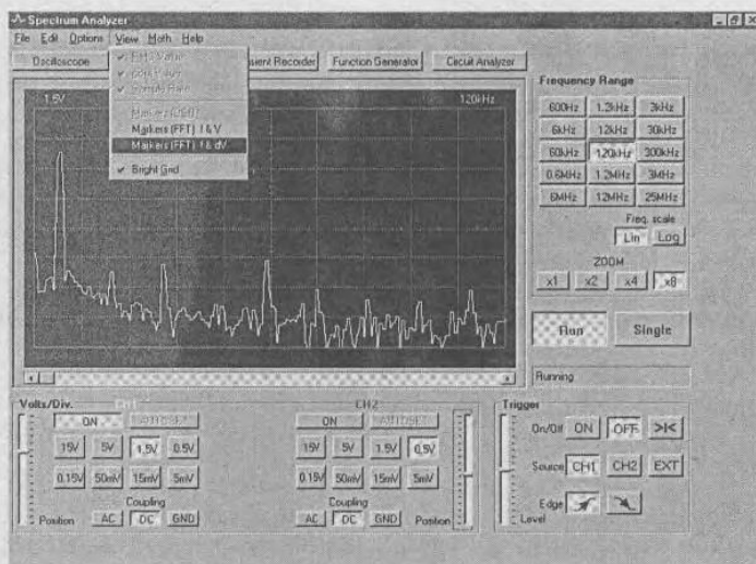
Рис. 4.7. Окно виртуального фурье-анализатора приставки PCS500
