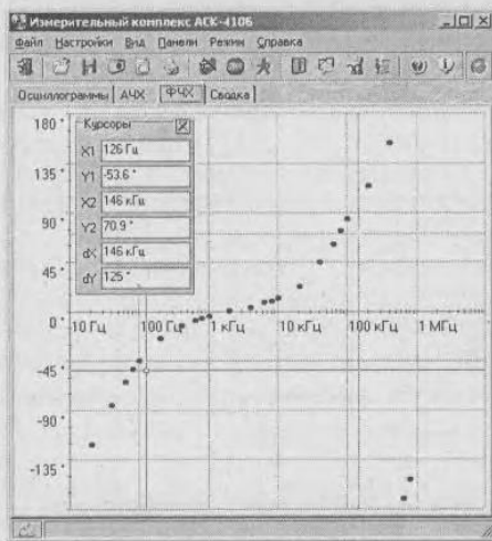
Рис. 6.74. Представление фазочастотной характеристики
