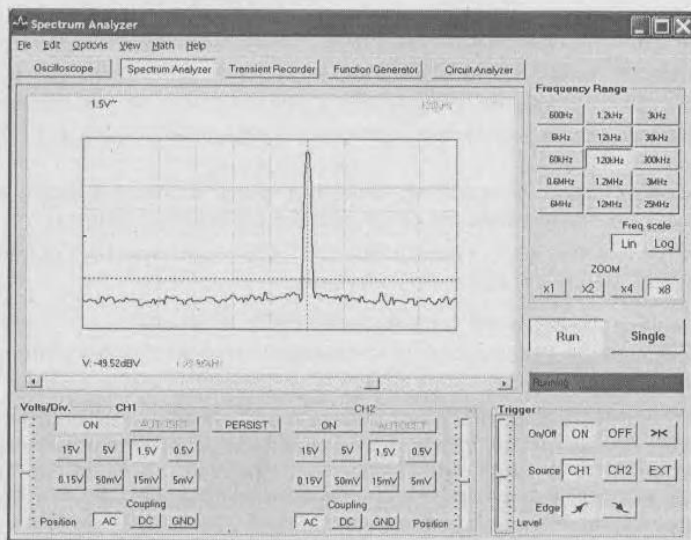
Рис. 6.35. Спектр синусоидального сигнала с частотой 100 кГц
