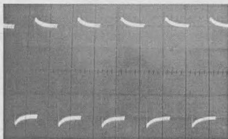
Рис. 5.10. Осциллограммы меандра при перекомпенсации делителя
