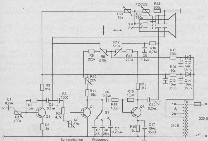
Рис. 2.4. Схема электронного осциллографа на трех транзисторах
