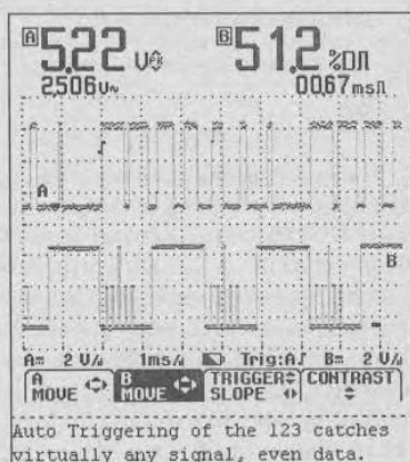
Рис. 3.44. Дисплей скопметра Fluke 123
