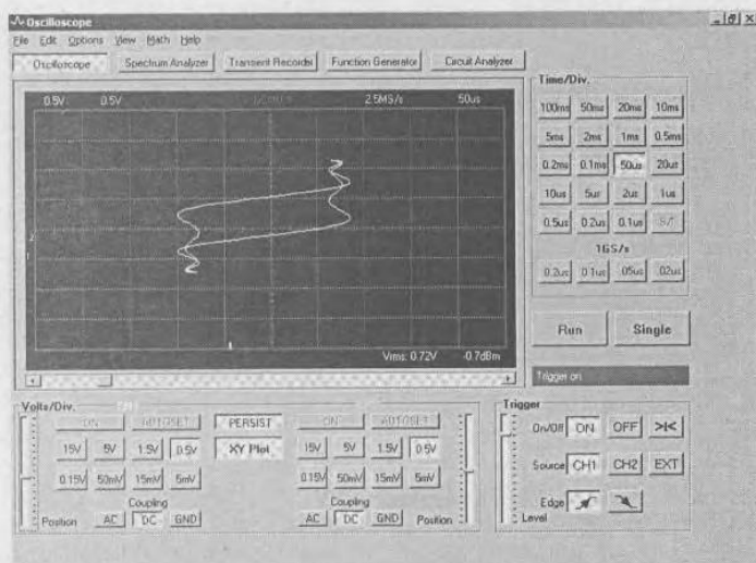
Рис. 6.11. Пример работы в режиме XY
