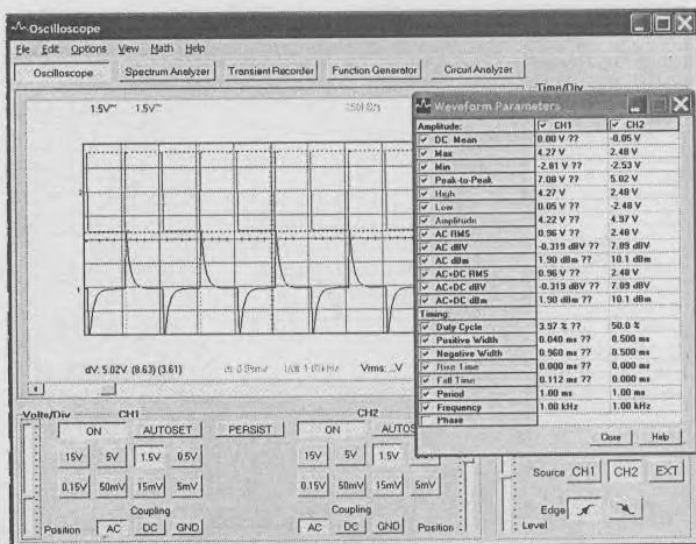
Рис. 6.23. Испытание дифференцирующей RC-цепи средствами лаборатории PC-Lab 2000
