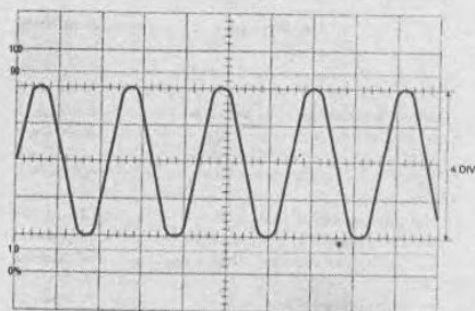
Рис. 5.18. Измерение двойного размаха синусоидального напряжения
