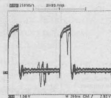
Рис. 5.71. Пример работы осциллографа с цифровым люминофором в режиме накопления осциллограмм
