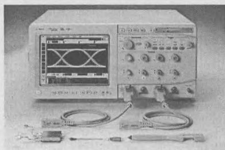
Рис. 3.38. Цифровой 12-гигагерцевый осциллограф DSO81304A
