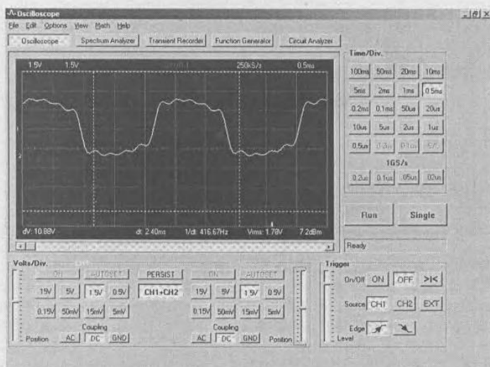
Рис. 6.9. Пример работы в режиме CH1 + CH2
