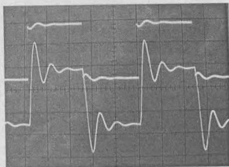
Рис. 5.41. Переходные процессы в LRC -цепи
