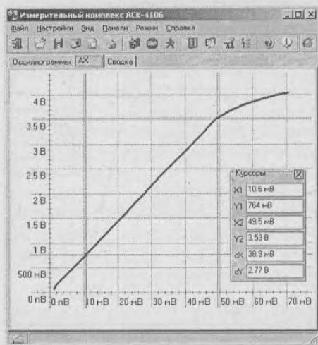
Рис. 6.73. Представление амплитудной (передаточной) характеристики
