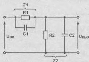
Рис. 5.7. Схема компенсированного делителя осциллографа
