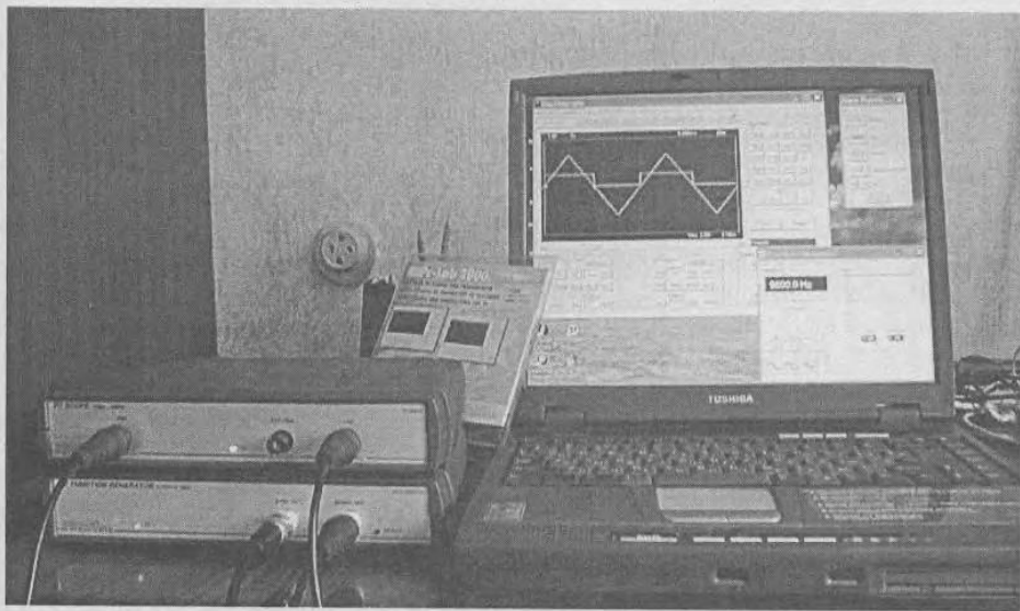
Рис. 4.13. Внешний вид компьютерной измерительной системы на базе виртуальных приборов и мобильного компьютера — ноутбука Satellite 1800-314 корпорации Toshiba
