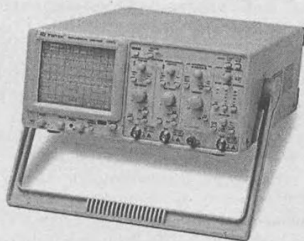
Рис. 2.22. Универсальный 200-мегагерцевый осциллограф GOS-6103
