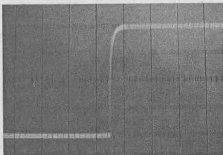
Рис. 5.12. Наблюдение фронта импульса от тестера
