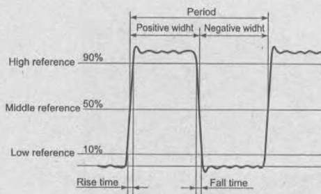
Рис. 4.24. К определению основных временных параметров импульсного сигнала
