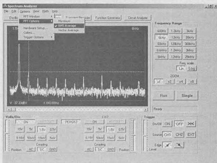
Рис. 4.25. Работа анализатора спектра в режиме запоминания спектрограмм
