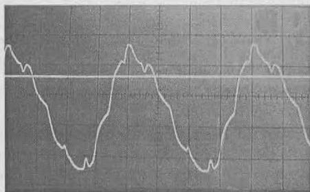
Рис. 5.2. Искраженная синусоида при пробе рукой
