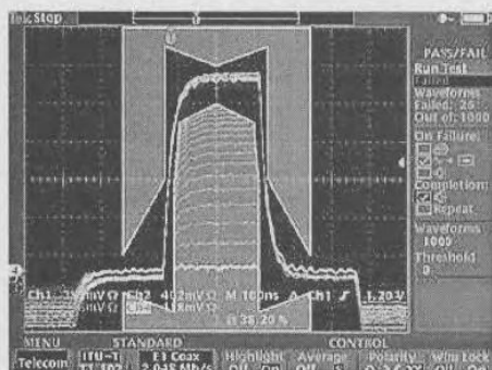
Рис. 3.65. Оциллограмма тестирования коммуникационной системы с помощью осциллографа серии TDS3000B
