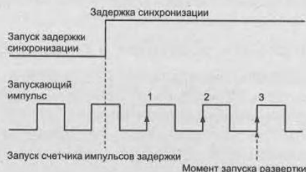
Рис. 5.66. Временные диаграммы запуска развертки по событию
