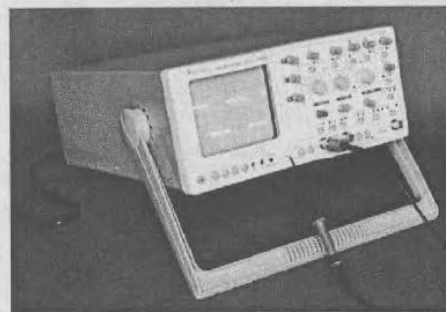
Рис. 2.9. Сервисный универсальный осциллограф С1-160
