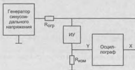
Рис. 5.29. Схема характериографа для снятия вольт-амперных характеристик двухполюсников
