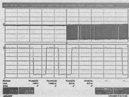
Рис. 5.48. Просмотр части изображения (нижняя осциллограмма) из общего изображения (верхняя осциллограмма), хранящегося в памяти (развертка 5 мс, растянутый фрагмент 1 мкс)
