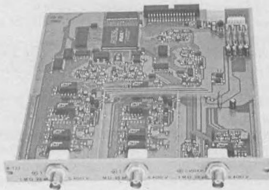
Рис. 4.29. Внешний вид осциллографа-платы В-121
