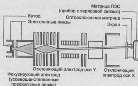
Рис. 2.31. Устройство конвертирующей ЭЛТ со сканирующей ПЗС-матрицей
