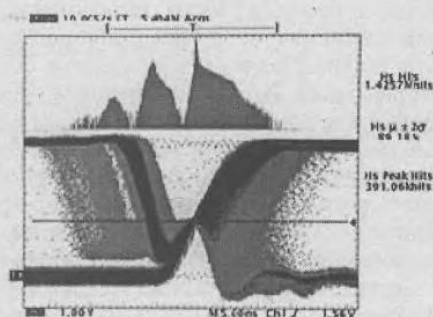
Рис. 5.69. Осциллограмма сложного нестабильного процесса с гистограммой интенсивности
