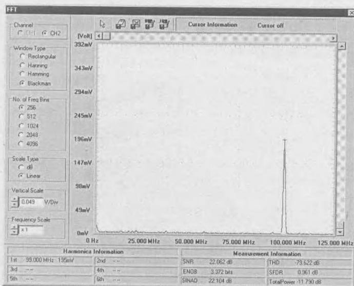
Рис. 4.39. Окно виртуального анализатора спектра приставки SDS200
