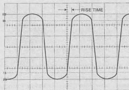
Рис. 5.21. Определение времени нарастания сигнала с выхода ограничителя
