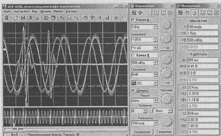
Рис. 6.54. Окно осциллографа-анализатора комбинированного прибора АСК-4106
