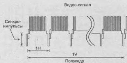
Рис. 5.17. Упрощенный вид телевизионного сигнала
