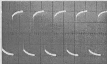
Рис. 5.9. Осциллограммы меандра при недокомпенсации искажений делителя
