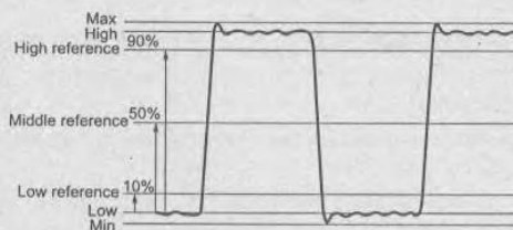
Рис. 4.23. К определению амплитудных параметров импульсного сигнала
