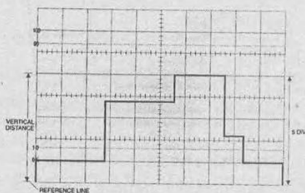
Рис. 5.19. Измерение параметров сложного импульса
