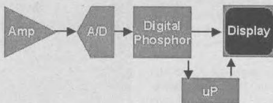
Рис. 5.68. Упрощенная функциональная схема осциллографа с цифровым люминофором
