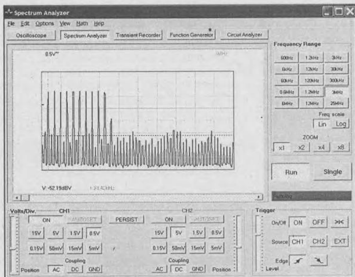
Рис. 6.45. Спектрограмма сигнала \sin(t)/t
