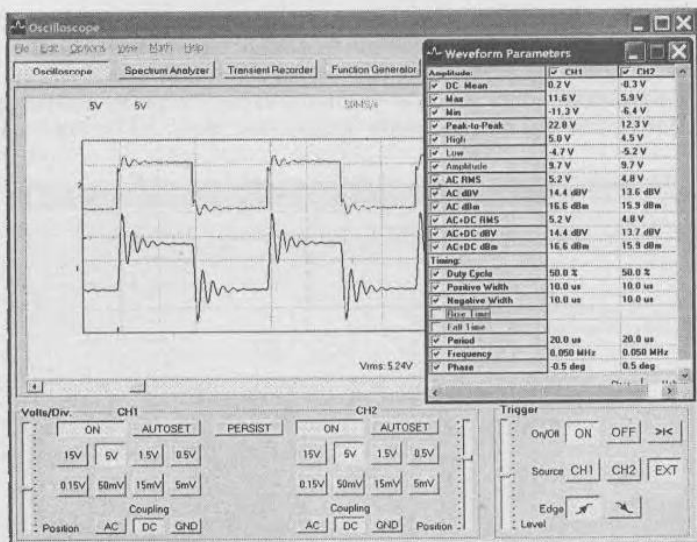
Рис. 6.29. Осциллограммы реакции LRC-цепочки на импульс — меандр
