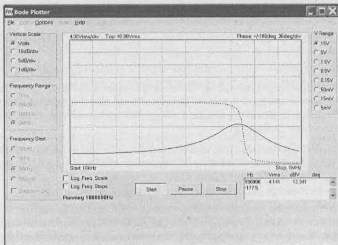
Рис. 6.47. Построение АЧХ и ФЧХ колебательного LRC-контура
