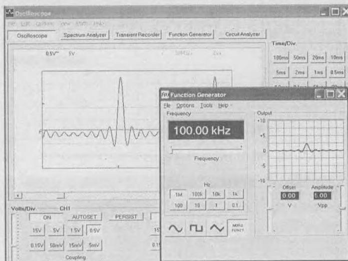
Рис. 6.44. Вывод и осциллограмма импульса вида \sin(t)/t
