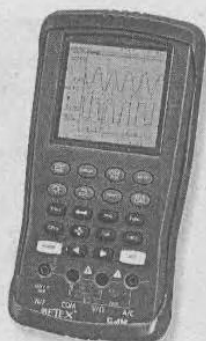
Рис. 3.58. Портативный мультиметр-осциллограф MS-2000 фирмы METEX
