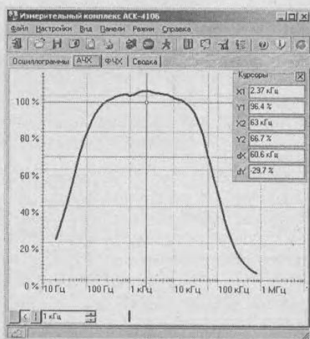
Рис. 6.72. Окно просмотра амплитудно-частотной характеристики
