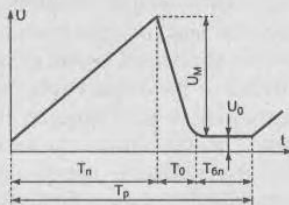
Рис. 1.20. Пилообразное напряжение развертки
