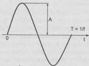
Рис. 1.1. Период синусоидального колебания (сигнала)
