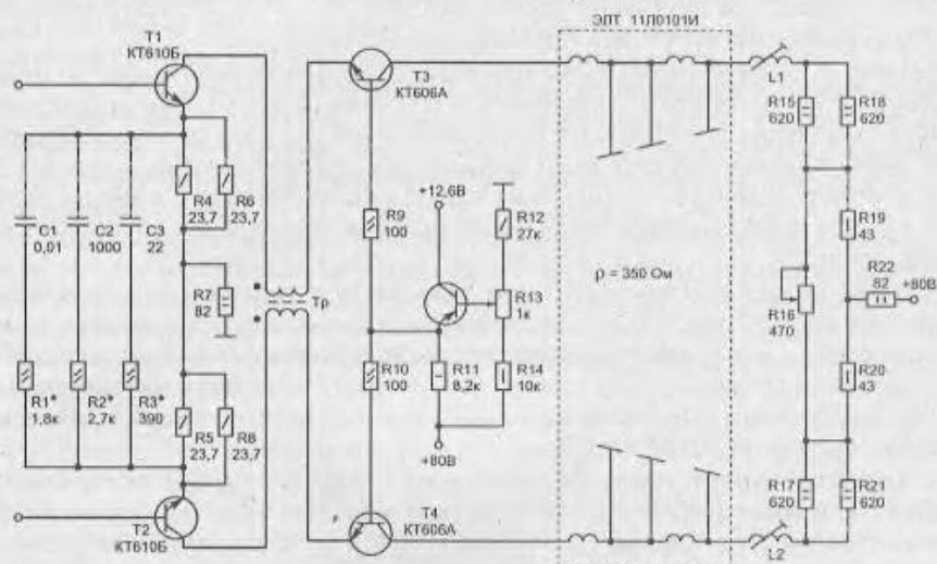
Рис. 1.19. Оконечный усилитель вертикального отклонения осциллографа СГ-71
