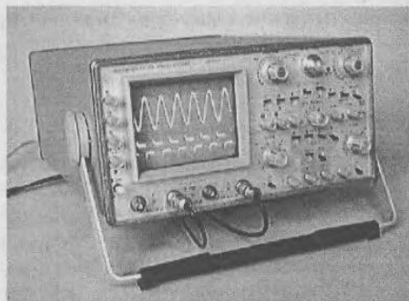
Рис. 2.10. Универсальный 4-канальный осциллограф С1-126
