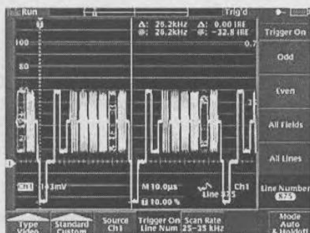
Рис. 3.66. Оциллограмма телевизионного сигнала на экране осциллографа серии TDS3000B
