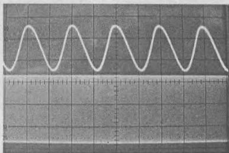
Рис. 5.32. Подготовка к наблюдению амплитудно-модулированного сигнала
