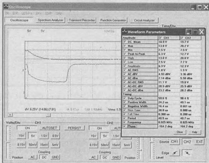
Рис. 6.33. Осциллограммы напряжений на конденсаторе C и коллекторе T1 при длительности развертки 2 мкс и окно вывода результатов автоматических вычислений
