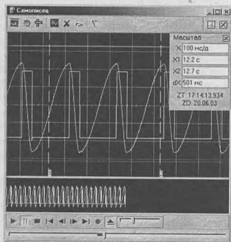
Рис. 6.63. Работа осциллографа в режиме самописца
