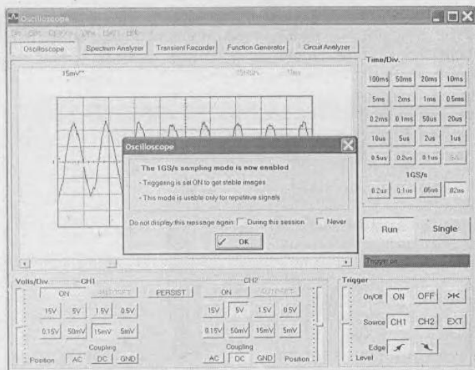
Рис. 6.15. Переход к осциллографированию с высокой частотой выборки
