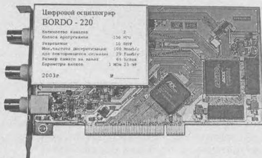
Рис. 4.32. Цифровой осциллограф — PCI-плата BORDO 221
