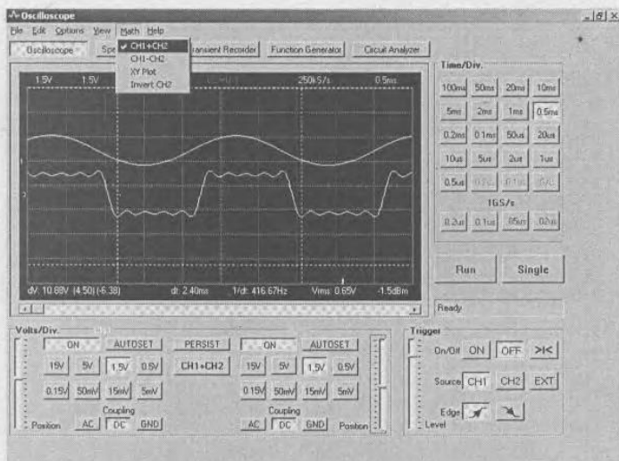
Рис. 6.8. Пример установки режима CH1 + CH2
