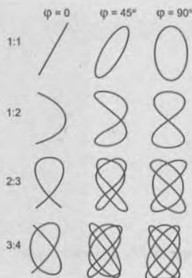
Рис. 5.28. Фигуры Лиссажу при сравнении кратных частот
