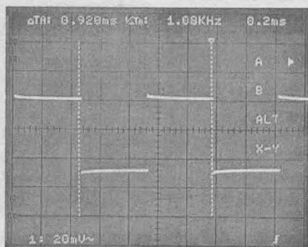
Рис. 5.43. Пример курсорного измерения периода колебаний
