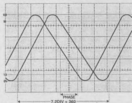
Рис. 5.20. Измерение периода синусоидального сигнала и фазы
