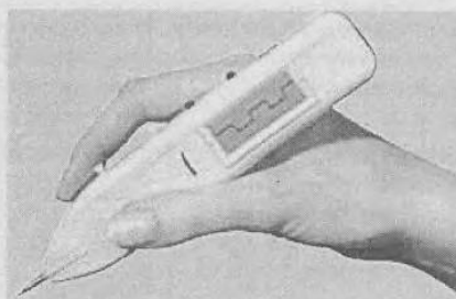
Рис. 3.42. Минископ (осциллограф-щуп) АСК-4011
