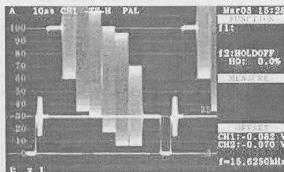
Рис. 2.36. Осциллография телевизионных сигналов
