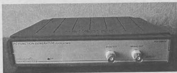
Рис. 4.8. Приставка — функциональный генератор PCG10 (вид спереди)
