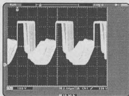
Рис. 5.75. Осциллографирование непрерывно изменяющихся импульсов
