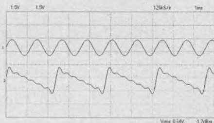
Рис. 4.17. Рисунок — осциллограммы с двух каналов осциллографа
