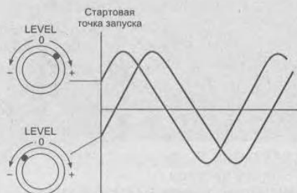
Рис. 5.15. Изменение уровня запуска развертки при синусоидальном сигнале
