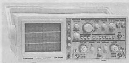
Рис. 2.28. Аналоговый осциллограф АСК-24020 с встроенным функциональным генератором
