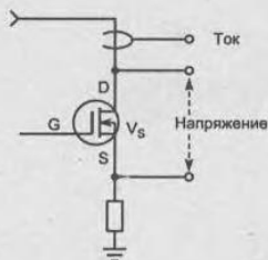
Рис. 5.73. Ключ на мощном полевом транзисторе — основной компонент преобразовательных устройств
