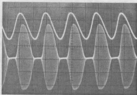
Рис. 5.34. Иллюстрация перемодуляции
