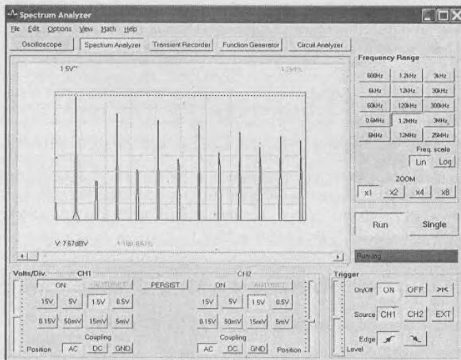
Рис. 6.43. Спектр треугольных импульсов
