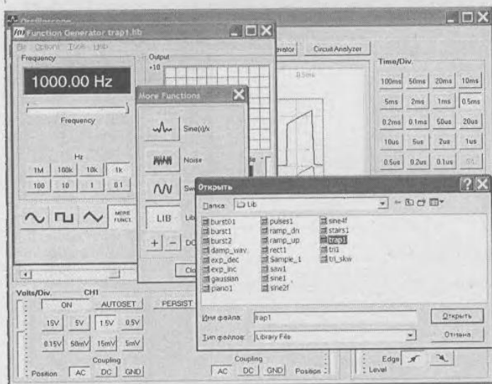
Рис. 6.27. Загрузка в функциональный генератор файла trap1.lib
