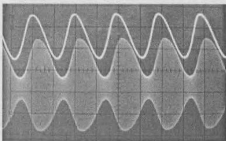
Рис. 5.33. Наблюдение модулирующего и модулированного сигналов
