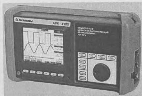
Рис. 3.25. Внешний вид цифрового запоминающего осциллографа АСК-2122
