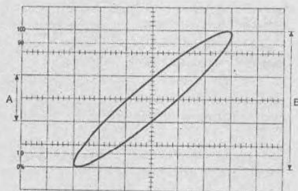
Рис. 5.25. К измерению фазового сдвига двух синусоидальных сигналов
