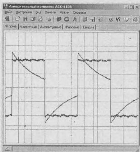
Рис. 6.71. Представление форм исследуемых напряжений
