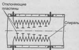
Рис. 1.10. Широкополосная отклоняющая система в виде линии передачи
