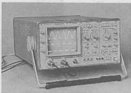
Рис. 2.13. Универсальный осциллограф С1-157 (100 МГц)
