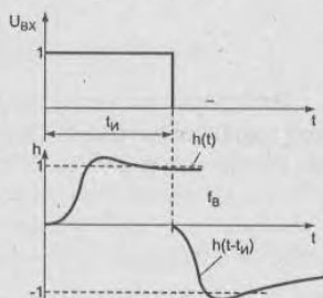
Рис. 1.15. Переходные характеристики усилителя
