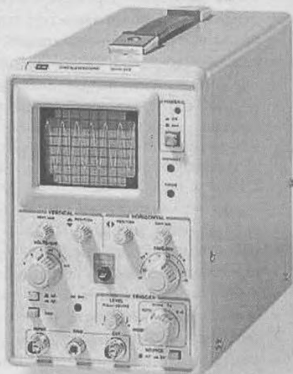
Рис. 2.15. Универсальный малогабаритный осциллограф GOS-310
