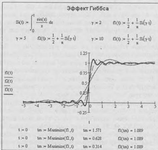
Рис. 1.4. Иллюстрация к возникновению эффекта Гиббса
