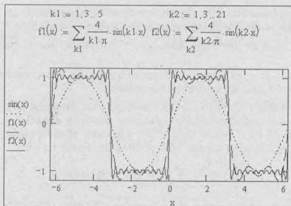
Рис. 1.2. Пример гармонического синтеза прямоугольных импульсов — меандра
