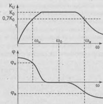
Рис. 1.13. Амплитудно-частотная и фазочастотная характеристики усилителя
