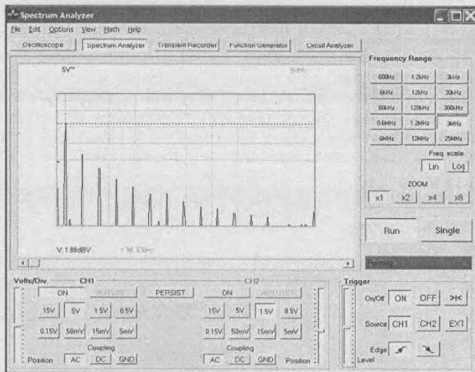
Рис. 6.42. Спектр прямоугольного импульса с заполнением, 10%
