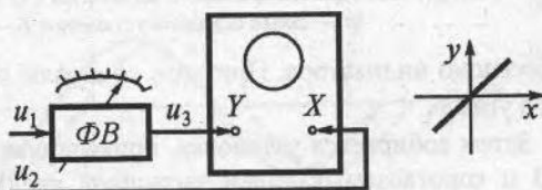
Рис. 9.6. К определению фазового сдвига компенсационным методом
