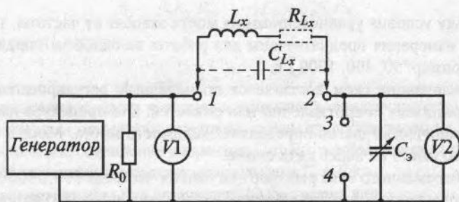
Рис. 12.8. Упрощенная структурная схема куметра
