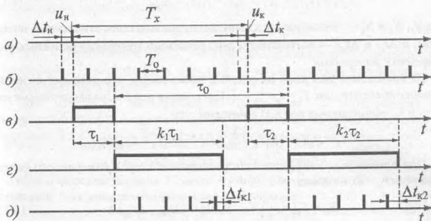
Рис. 8.9. Измерение временного интервала методом интерполяции:
