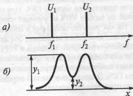
Рис. 11.6. Диаграммы к определению разрешающей способности анализатора спектра: а — спектр сигнала; б — эюры спектров на экране
