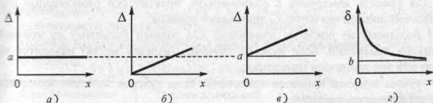
Рис. 2.12. Виды погрешностей средств измерений:
