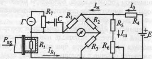
Рис. 10.5. Схема уравновешенного моста с терморезистором
