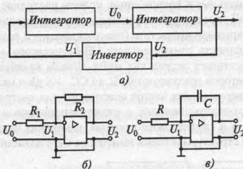
Рис. 6.6. Структурные схемы колебательного звена: а — электронная модель; б — усилительная; в — интегрирующая
