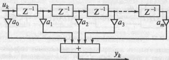
Рис. 11.13. Структурная схема нерекурсивного цифрового фильтра
