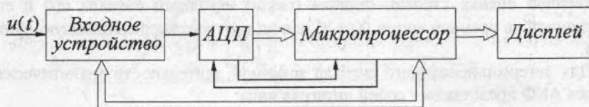
Рис. 13.7. Микропроцессорный измеритель характеристик распределения вероятностей
