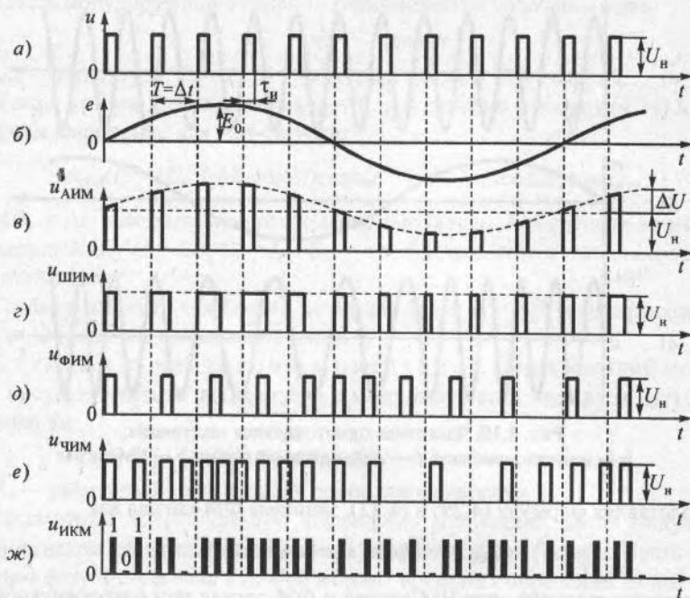
Рис. 4.11. Импульсная модуляция:
