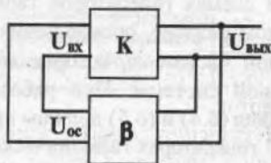
Рис. 6.1. Обобщенная структурная схема генератора
