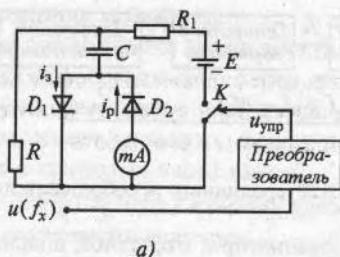
Рис. 8.6. Конденсаторный частотомер: а — структурная схема; б — временные диаграммы к схеме
