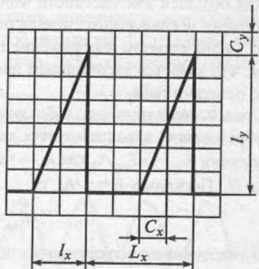
Рис. 7.14. Определение параметров сигнала с помощью масштабной сетки
