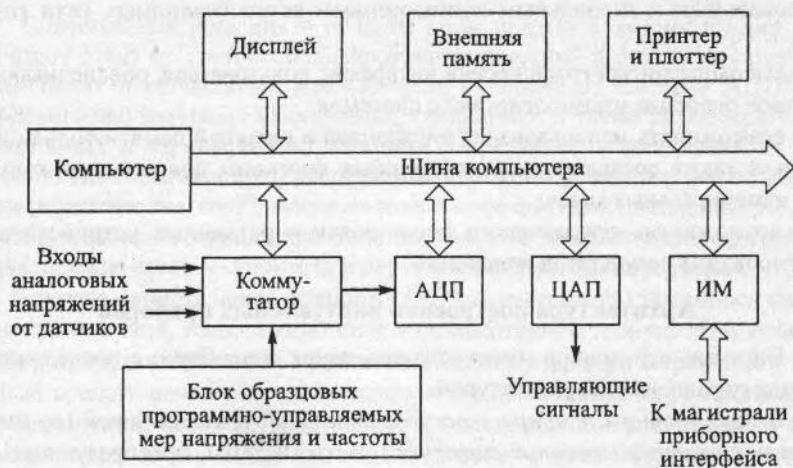
Рис. 14.2. Обобщенная структурная схема виртуального прибора
