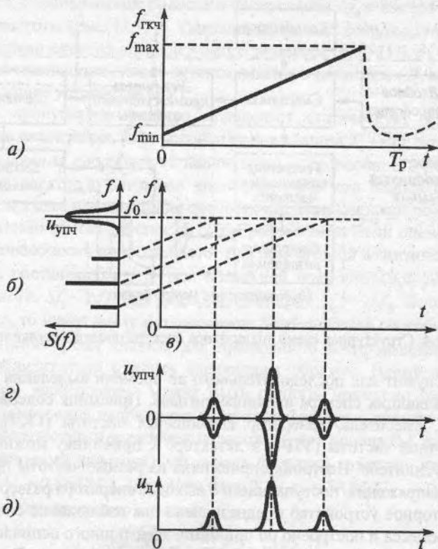
Рис. 11.5. Сигналы в анализаторе спектра последовательного типа:
