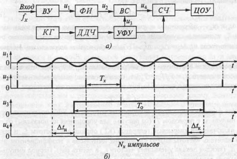
Рис. 8.7. Цифровой частотомер:
