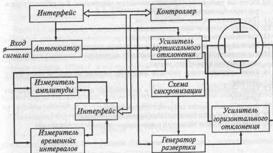
Рис. 7.19. Упрощенная структурная схема цифрового осциллографа
