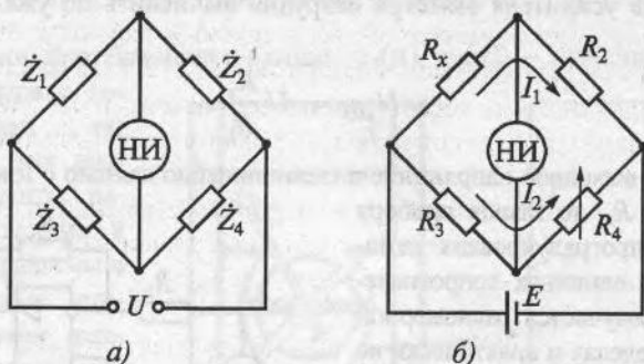
Рис. 12.5. Схемы четырехплечих мостов: а — обобщенная; б — для измерения активных сопротивлений
