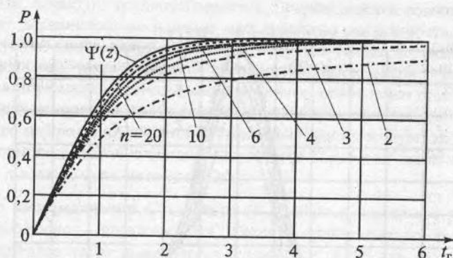
Рис. 2.7. Графики вероятностей P(-t_r < t < t_r)_n при законе распределения Стьюдента для различных значений n и функции \Psi(z)
