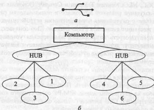
Рис. 14.9. Топология интерфейса USB:
