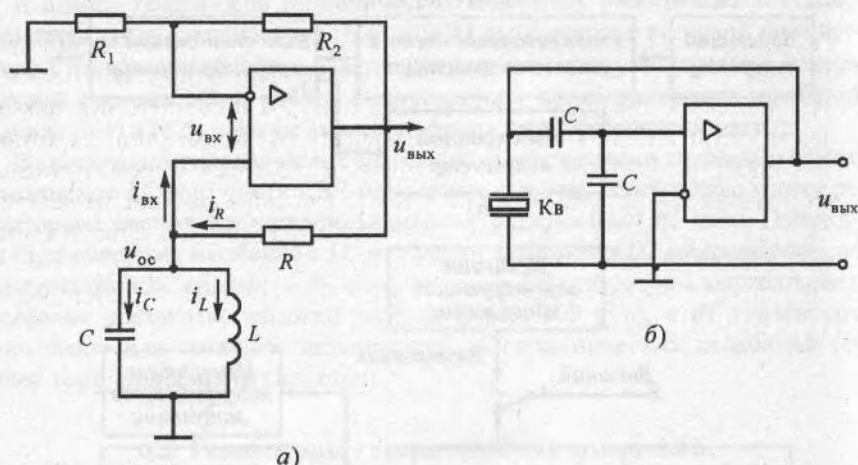
Рис. 6.3. LC -генераторы на ОУ:
