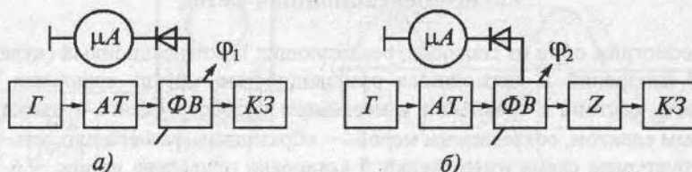
Рис. 9.7. Измерение фазового сдвига на СВЧ компенсационным методом: а — схема исходной установки; б — схема измерения
