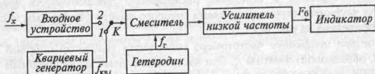
Рис. 8.4. Упрощенная структурная схема гетеродинного частотомера
