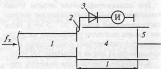
Рис. 8.3. Упрощенная структурная схема резонансного частотомера
