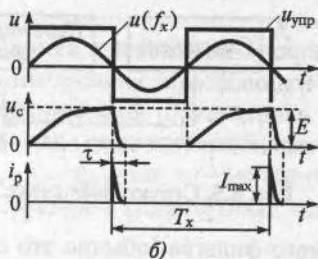
Рис. 8.6. Конденсаторный частотомер: а — структурная схема; б — временные диаграммы к схеме
