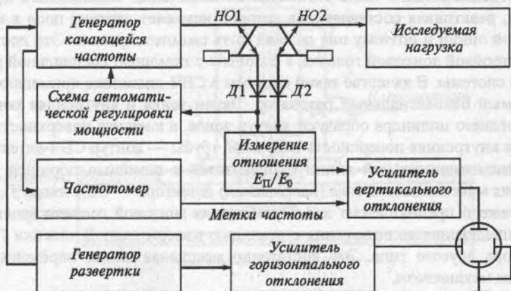
Рис. 12.21. Упрощенная структурная схема панорамного рефлекметра
