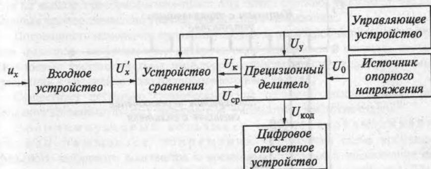
Рис. 5.12. Упрощенная структурная схема кодоимпульсного вольтметра
