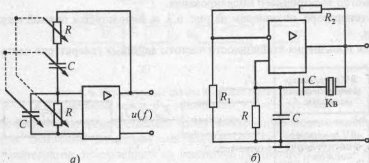
Рис. 6.4. Схемы RC -генераторов с мостом Вина:
