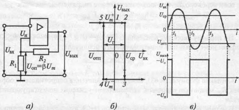
Рис. 4.29. Компаратор:
