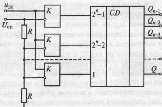
Рис. 4.32. Структурная схема параллельного АЦП
