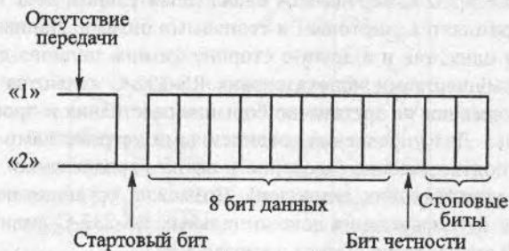
Рис.14.8. Формат данных RS-232-C
