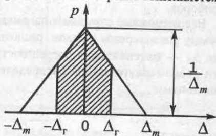
Рис. 2.9. Треугольный закон распределения
