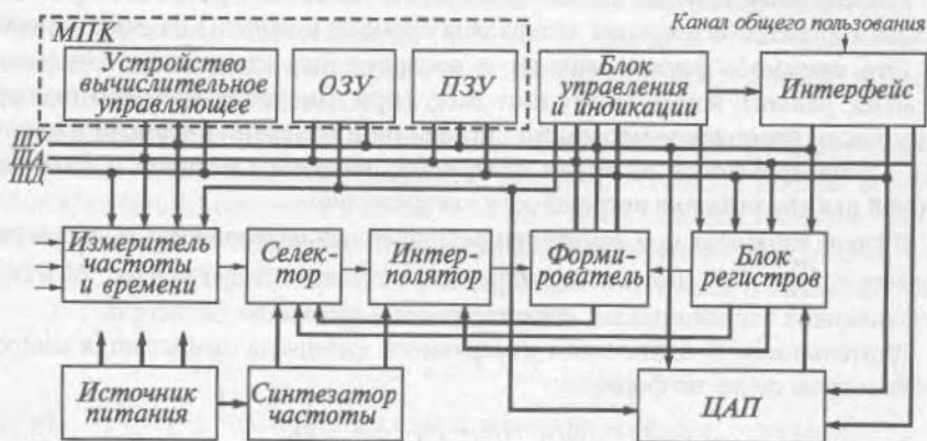
Рис. 8.10. Упрощенная структурная схема ИВИ с микропроцессором
