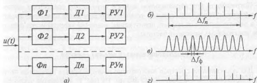
Рис. 11.3. Параллельный анализ спектра: а — структурная схема анализатора; б — исследуемый спектр; в — АЧХ фильтров; з — спектр на выходе анализатора
