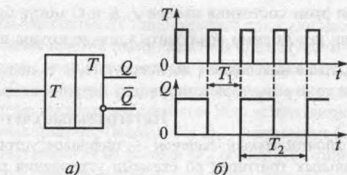
Рис. 4.20. T -триггер:
