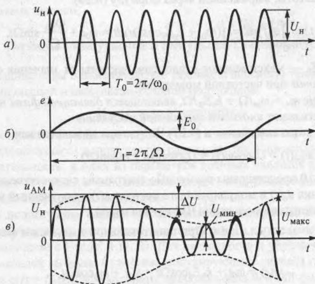
Рис. 4.9. Амплитудная модуляция:
