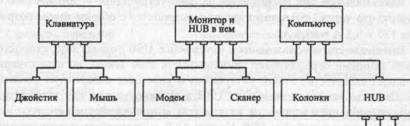
Рис. 14.10. Пример соединения периферийных устройств в USB-сеть
