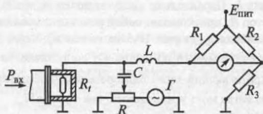
Рис. 10.4. Схема неуравновешенного моста
