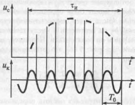
Рис. 7.15. Измерение интервалов времени с помощью калибровочных меток:
