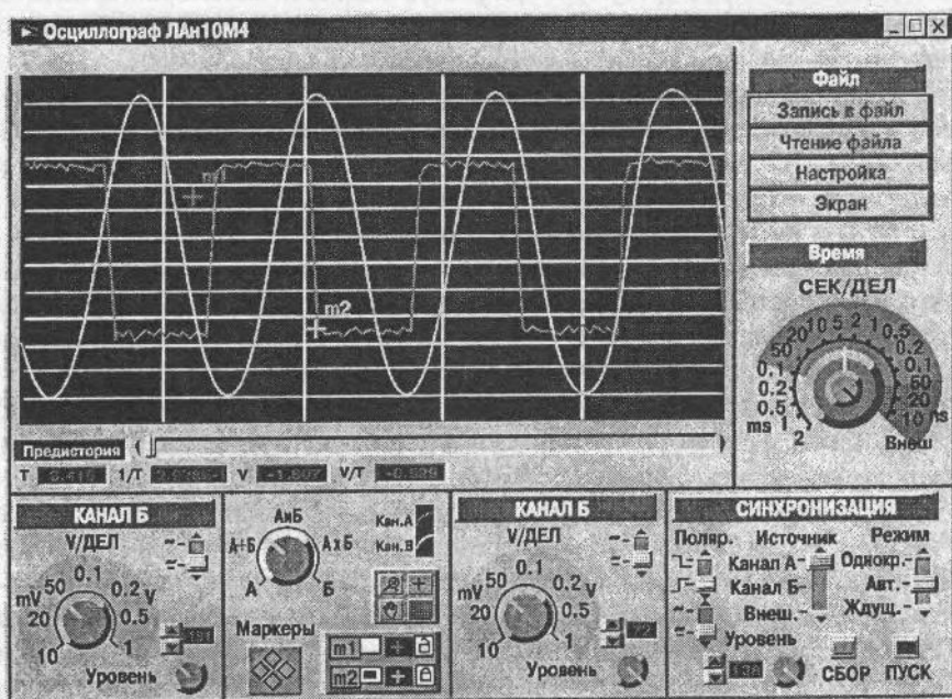
Рис. 14.3. Внешний вид программного интерфейса виртуального осциллографа
