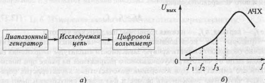
Рис. 12.15. К методу снятия АЧХ по точкам:
