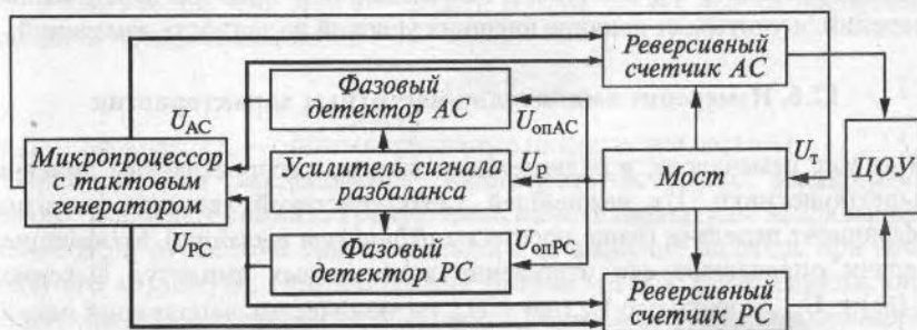
Рис. 12.13. Упрощенная структурная схема цифрового автоматического измерителя комплексного сопротивления с микропроцессором
