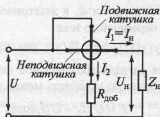
Рис. 10.1. Схема электродинамического ваттметра
