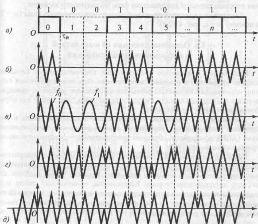
Рис. 4.12. Виды цифровой модуляции двоичным кодом: а — код; б — ИКМ-АМ; в — ИКМ-ЧМ; з — ИКМ-ФМ; д — ОФМ
