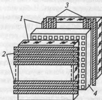
Рис. 7.11. Матричная индикаторная панель: 1 — стеклянные пластины; 2 — аноды; 3 — катоды; 4 — матрица
