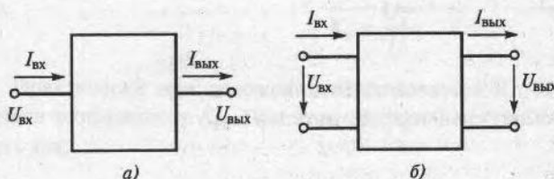
Рис. 12.1. Радиотехнические цепи: а — двухполосник; б — четырехполосник
