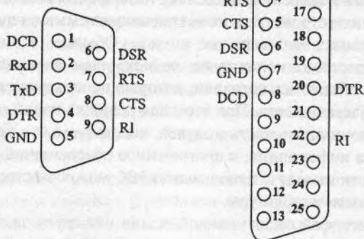
Рис. 14.6. Разъемы компьютера для подключения интерфейса RS-232-C
