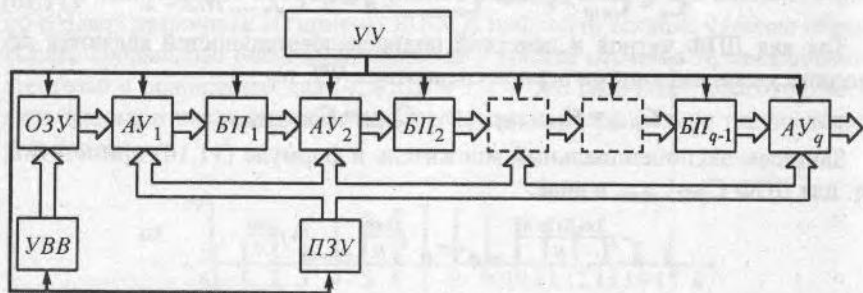
Рис. 11.9. Структурная схема анализатора с реализацией БПФ
