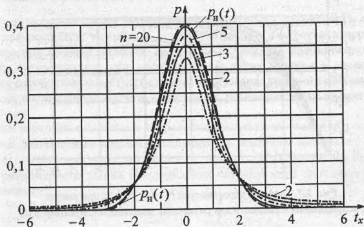
Рис. 2.6. Графики распределения Стюдента p(t_x)_n для различных n и нормированного нормального распределения p_n(t) при t = t_x
