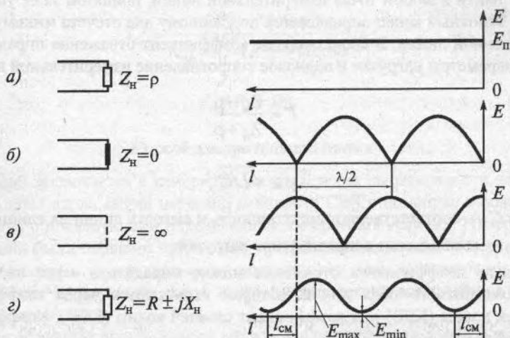
Рис. 12.19. Распределение поля вдоль измерительной линии в режимах: а — бегущей волны; б — короткого замыкания; в — холостого хода; г — смешанных волн
