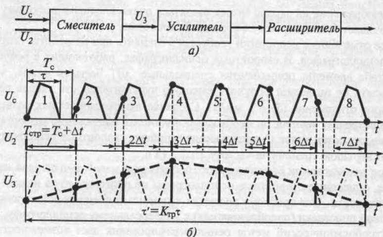
Рис. 7.13. Принцип работы преобразователя стробоскопического осциллографа: а — схема; б — временные диаграммы
