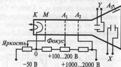
Рис. 7.6. Схема управления лучом ЭЛТ
