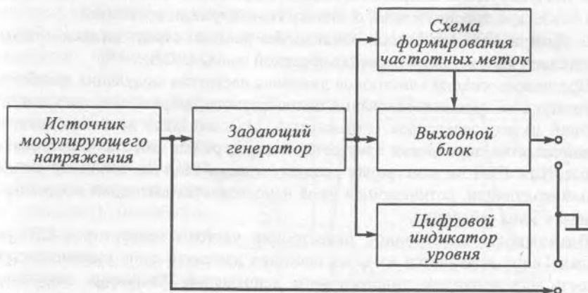
Рис. 6.9. Упрощенная структурная схема генератора качающейся частоты
