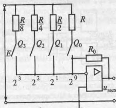
Рис. 4.30. Четырехразрядный ЦАП
