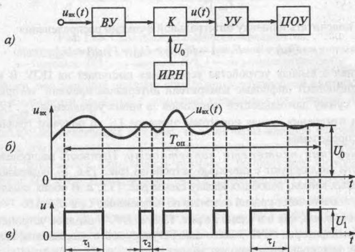
Рис. 13.5. Измерение функции распределения вероятностей: а — структурная схема; б — время пребывания реализации выше уровня анализа; в — импульсы на выходе компаратора
