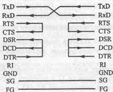
Рис. 14.7. Схема четырехпроводной линии связи для RS-232-C
