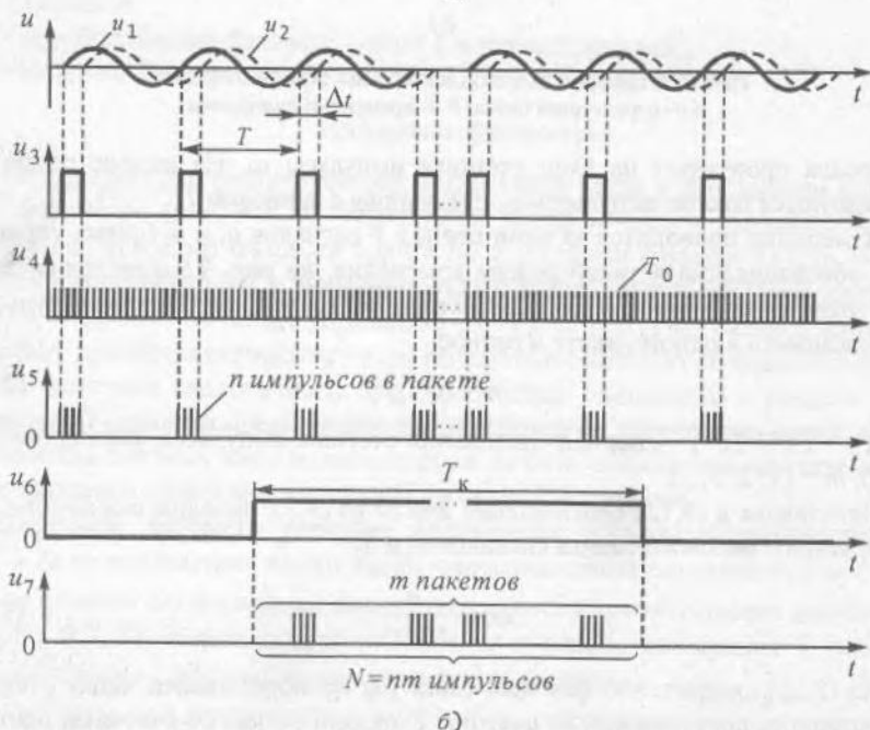
Рис. 9.10. Измерение сдвига фаз цифровым фазометром среднего значения: а — схема; б — эспоры к схеме
