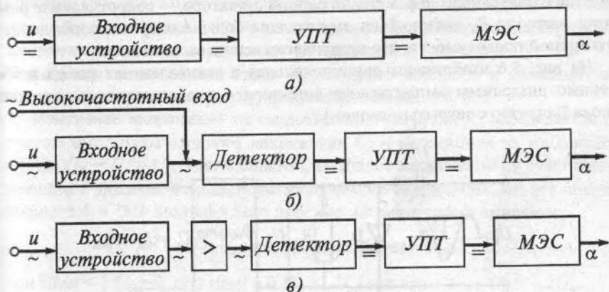
Рис. 5.5. Структурные схемы аналоговых электронных вольтметров: а — постоянного тока; б — напряжений большого уровня; в — милливольтметра (УПТ — усилитель постоянного тока; > — усилитель переменного тока; МЭС — магнитоэлектрическая система — стрелочный прибор)
