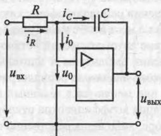
Рис. 7.9. Генератор развертки на ОУ
