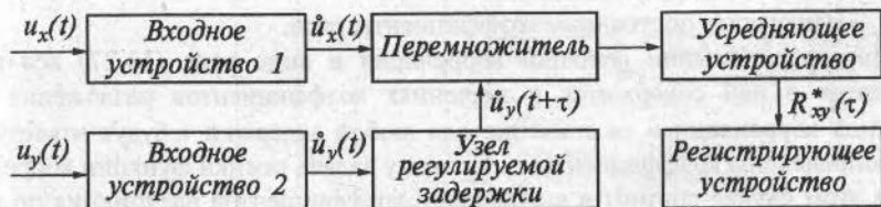
Рис. 13.9. Структурная схема коррелометра с перемножением
