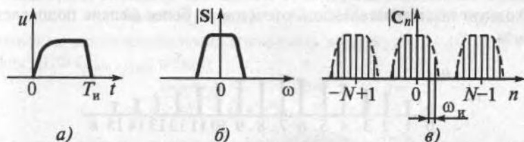
Рис. 11.7. Представление аналогового сигнала дискретным преобразованием Фурье: а — сигнал; б — спектр сигнала; в — ДПФ сигнала
