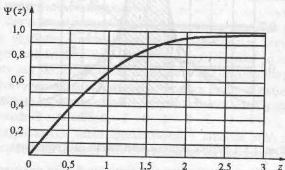
Рис. 2.4. График значений функции \Psi(z) для z \geq 0
