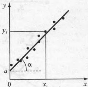
Рис. 3.2. Аппроксимация исследуемой зависимости
