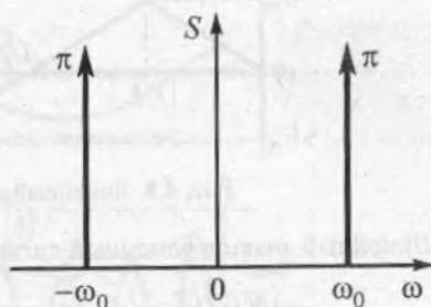
Рис. 4.6. Спектральная плотность гармонического сигнала
