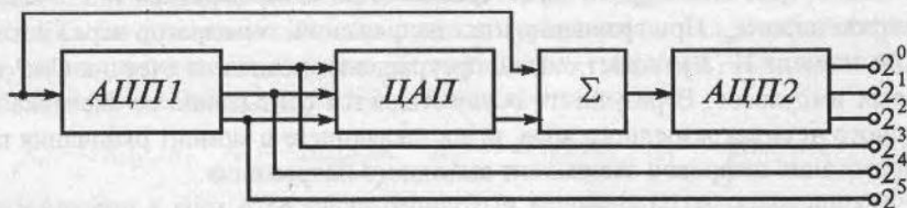
Рис. 4.33. Структурная схема последовательно-параллельного АЦП
