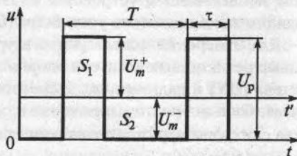
Рис. 5.17. Диаграммы к вольтметру с амплитудным преобразователем
