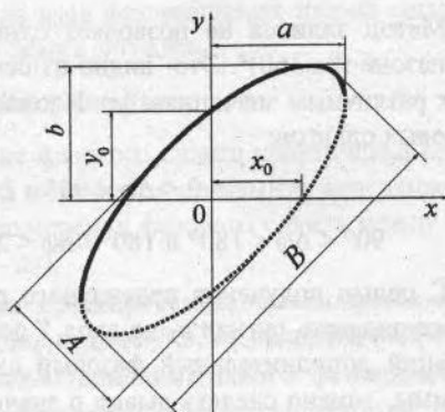
Рис. 9.3. К измерению разности фаз методом эллипса
